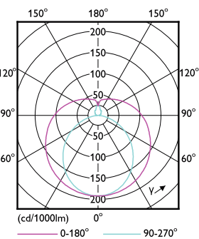
LEDtube MAS 26W G5 3700lm
