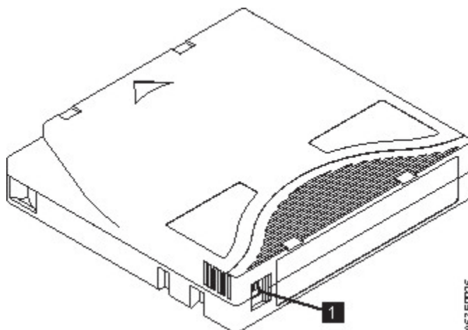
Figura 89. Posición del conmutador de protección contra grabación
