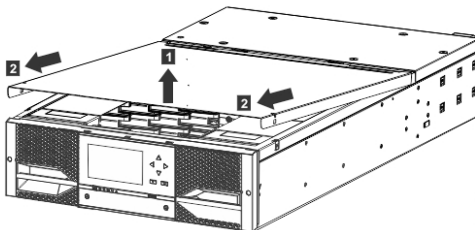
Figura 22. Retirada de la parte superior del módulo
