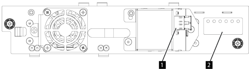
Figura 43. Puerto FC único de altura media
