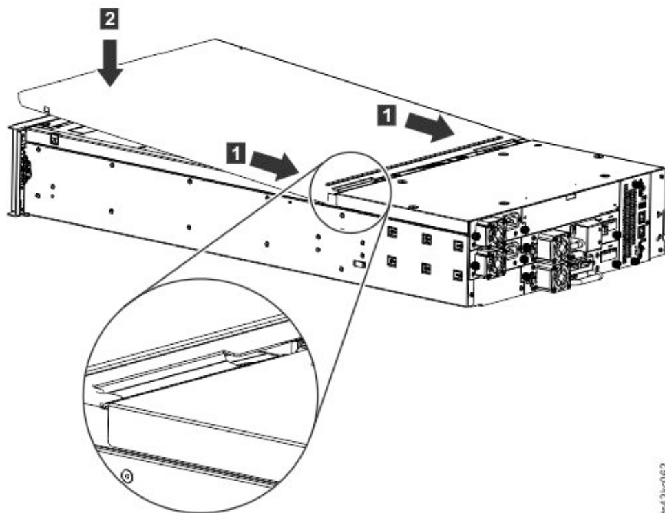
Figura 25. Bajada de la parte frontal de la cubierta superior
