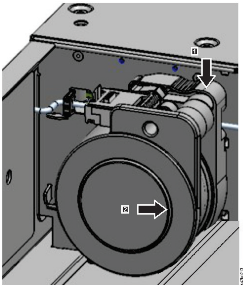
Figura 80. Desbloquee el mecanismo de spooling
