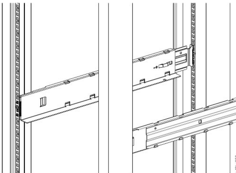
Figura 33. Rieles laterales instalados
