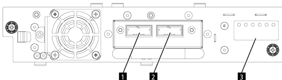
Figura 44. Puerto dual SAS de altura media
