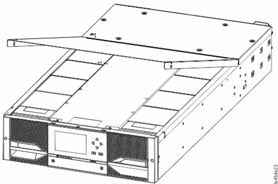
Figura 23. Este módulo se abre para mostrar el embalaje de espuma.
