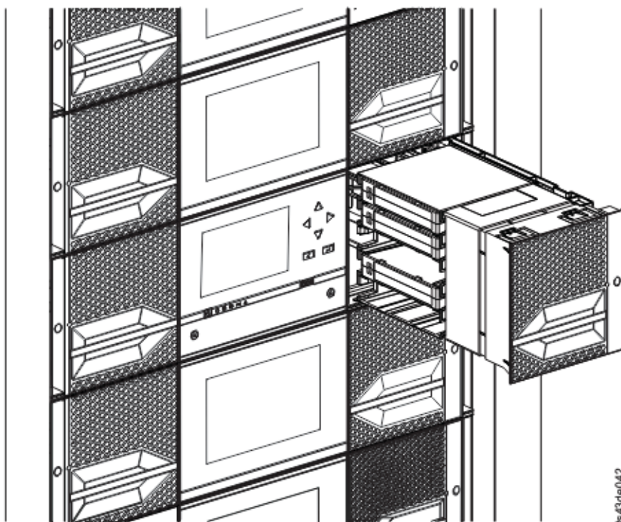
Figura 47. Estación de E/S abierta vista desde la izquierda
