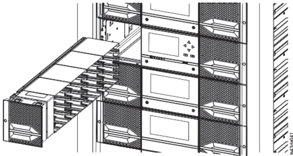
Figura 48. Cargador extraído
