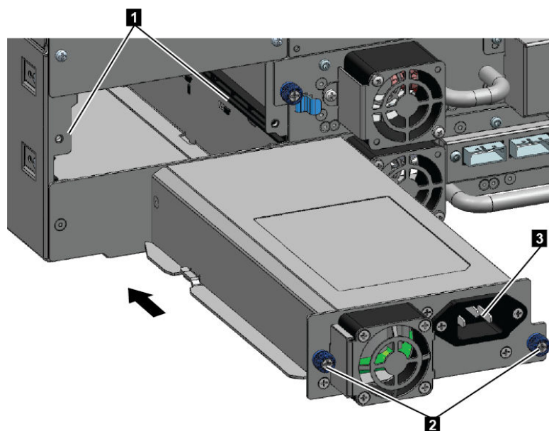
Figura 68. Deslizamiento de la nueva fuente de alimentación
