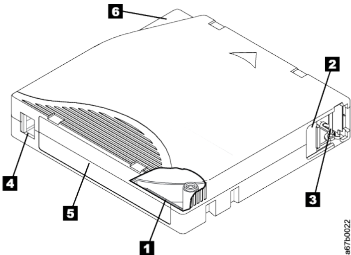
Figura 86. Cartucho de datos LTO Ultrium
