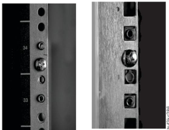
Figura 31. Ubicaciones de conector correctas
