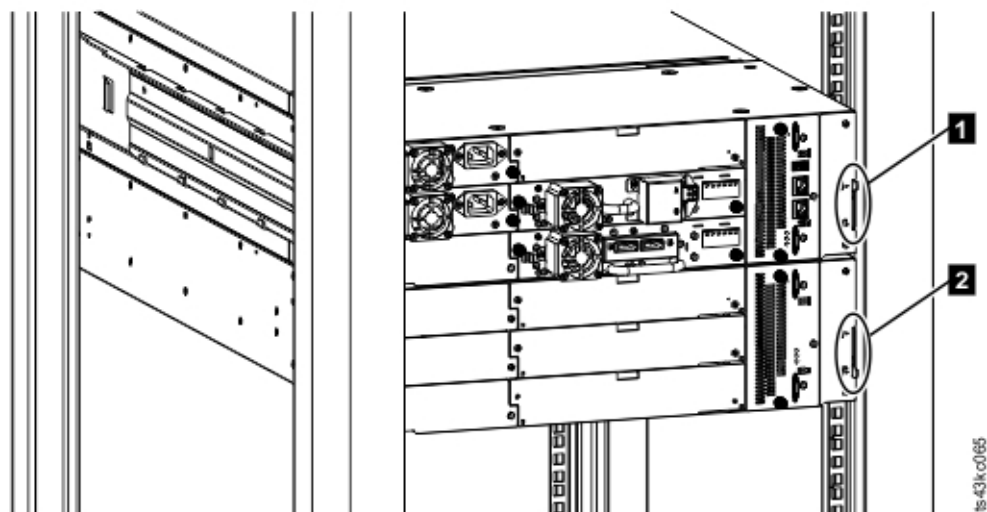
Figura 40. Dos módulos del bastidor, vistos desde la parte posterior
