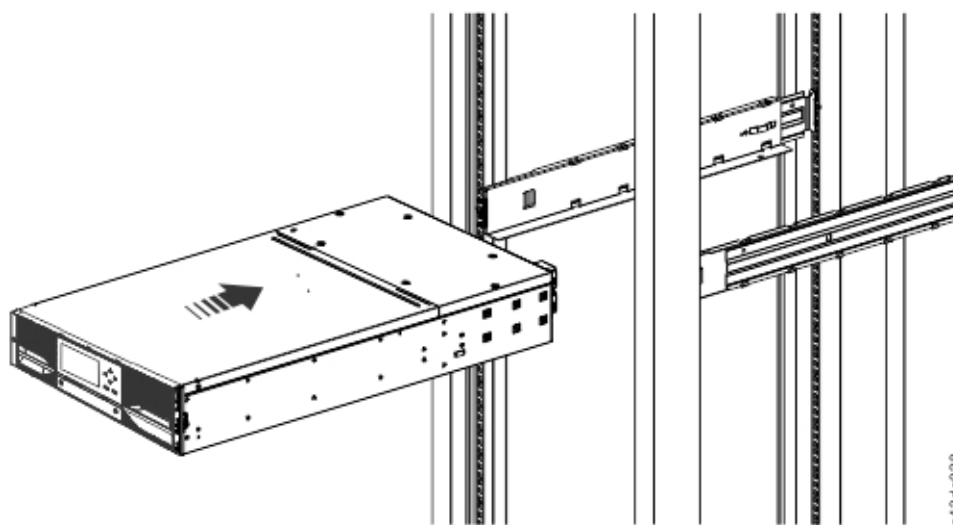
Figura 34. Deslizamiento de la biblioteca en el bastidor
