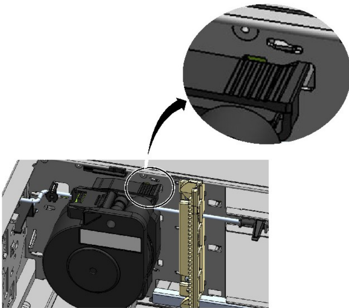
Figura 81. Mecanismo de spooling desbloqueado - vista ampliada
