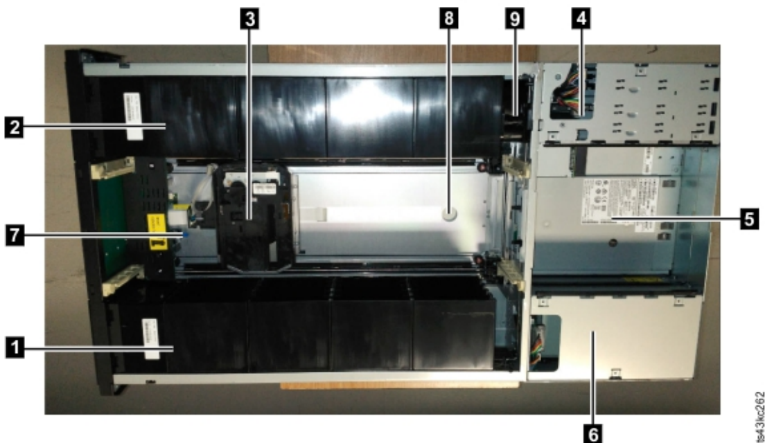
Figura 58. Vista interna de la biblioteca
