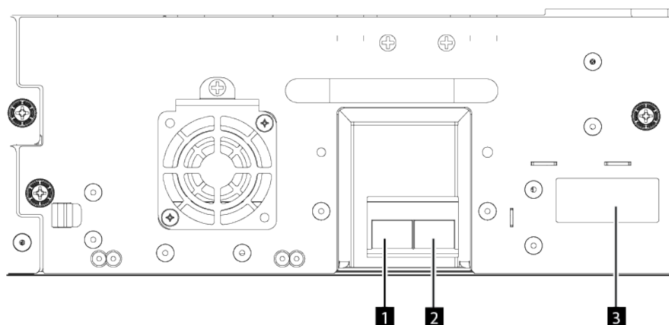
Figura 17. Puerto dual FC de altura completa
