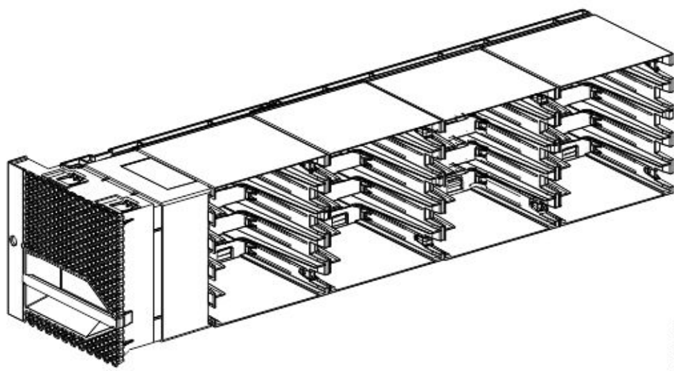
Figura 9. Cargador izquierdo
