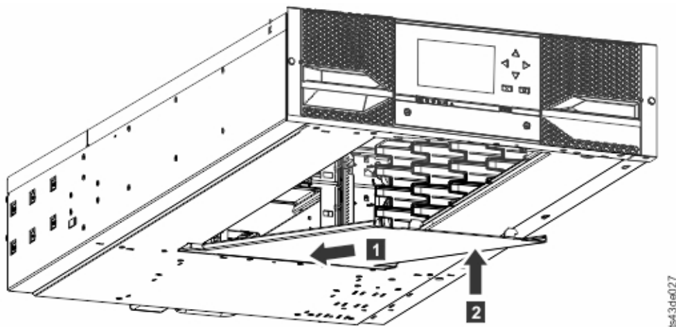
Figura 28. Levantamiento de la cubierta y bloqueo
