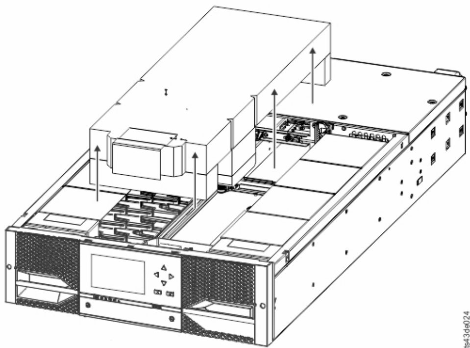
Figura 24. El embalaje de espuma se retira y se muestran los componentes internos - Módulo base.
