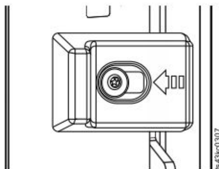
Figura 37. Bloqueo de palanca de alineación
