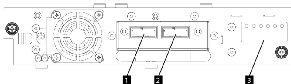
Figura 15. Puerto dual SAS de altura media
