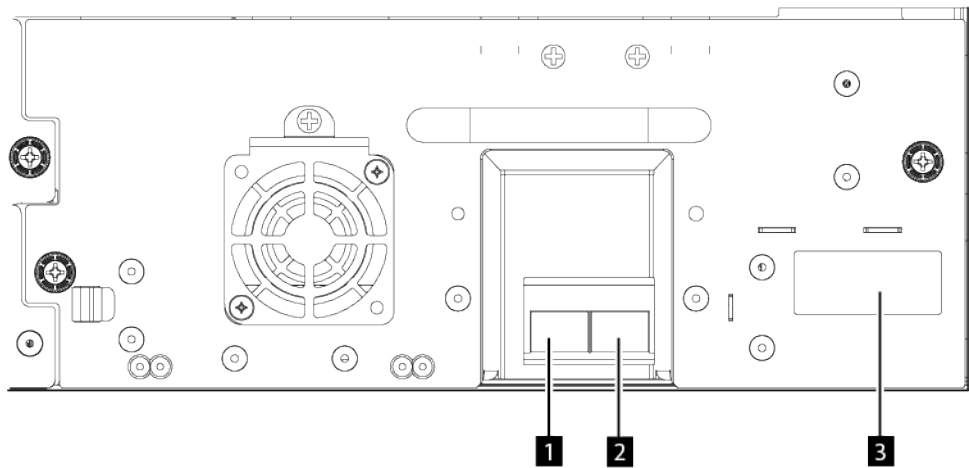
Figura 42. Puerto dual FC de altura completa
