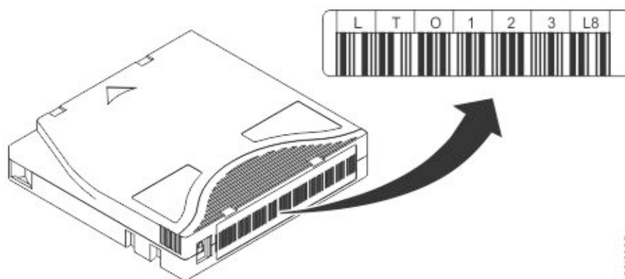
Figura 88. Etiqueta de código de barras de ejemplo en el cartucho de cintas LTO Ultrium
