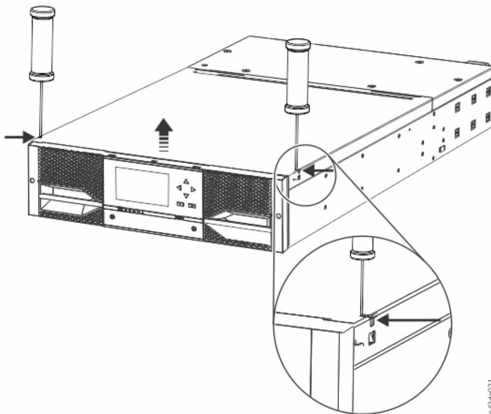
Figura 21. Apertura de la parte superior del módulo
