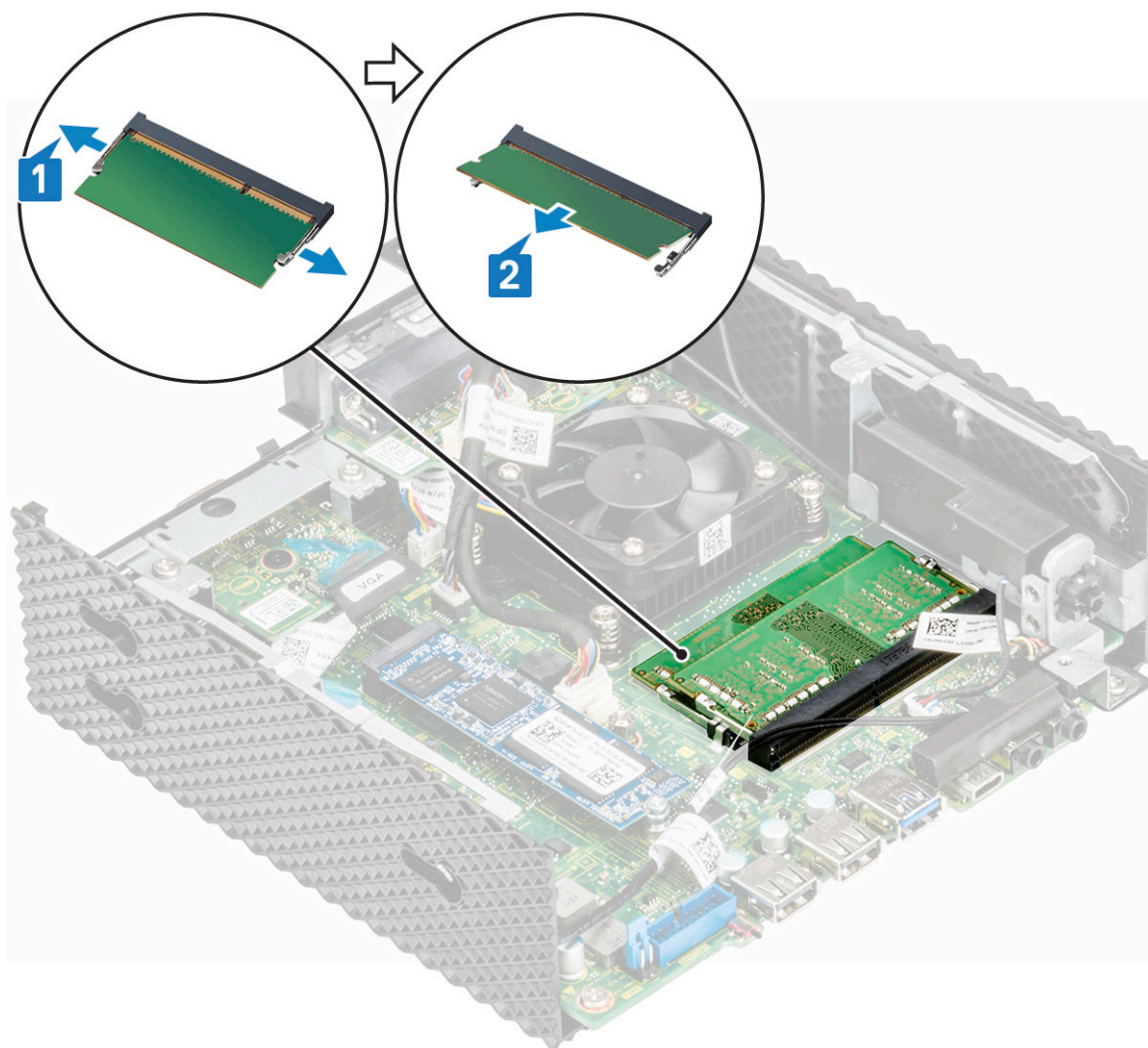
Figura 22. Rimuovere il modulo di memoria
