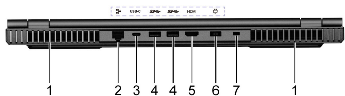
Figura 7. Vista posteriore - modelli da 15 pollici
