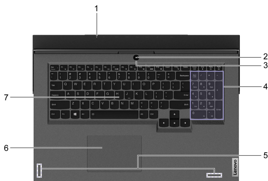
Figura 3. Vista base - modelli da 17 pollici
