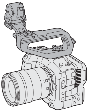
Configurazione con portamicrofono e maniglia
