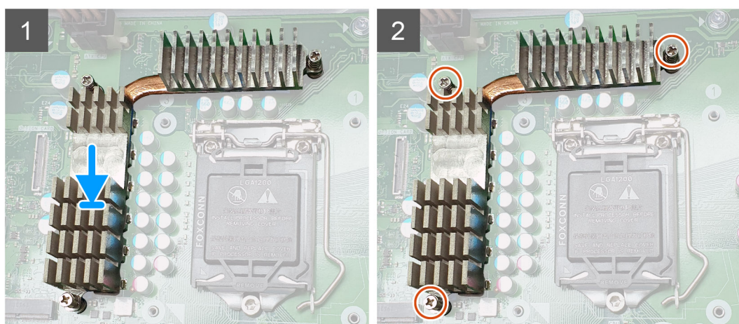
Figur 13. VR-kylflänsmontering för system som levereras med 125 W CPU
