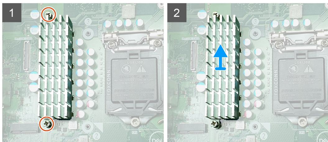
Figur 12. VR-kylflänsmontering för system som levereras med 65 W eller 80 W CPU
