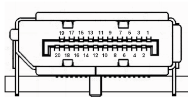
Cavo per segnale di visualizzazione a colori a 20 pin
