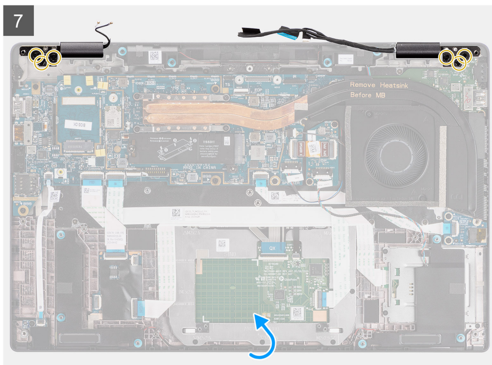
Afbeelding 3. De beeldscherm eenheid met WLAN- en WWAN-antenne
