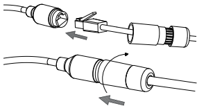
Рисунок 16: Крепление водонепроницаемого коннектора
