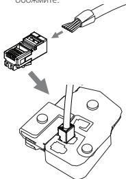
Рисунок 15: Крепление коннектора RJ-45
