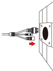
Figura 10: Fissaggio dei cavi
