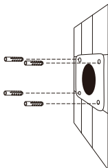
Figura 9: Acoplamiento de los anclajes de la pared
