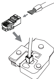
Figura 15: Collegamento del connettore RJ-45
