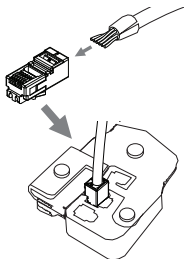
Abbildung 15: RJ-45-Stecker anbringen
