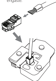
Figura 15: Acoplamiento del conector RJ-45
