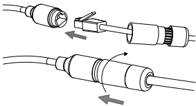
Figure 16 : Fixation du connecteur étanche
