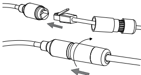
Figura 16: Acoplamiento del conector impermeable
