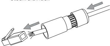
Abbildung 14: Kabel durchführen
