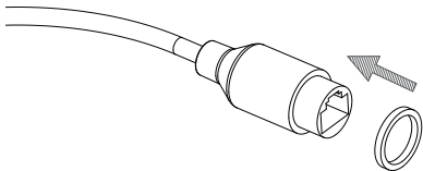
Рисунок 13: Установка уплотнительной прокладки
