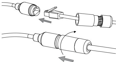
Рисунок 16: Крепление водонепроницаемого коннектора
