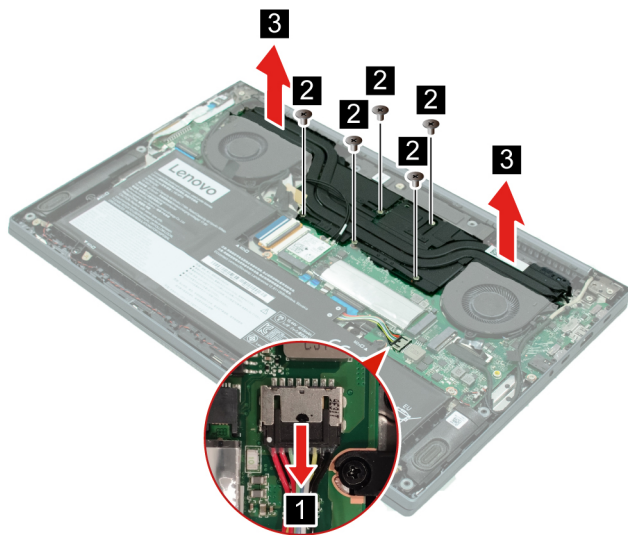
Figure 14. Remove the thermal module
