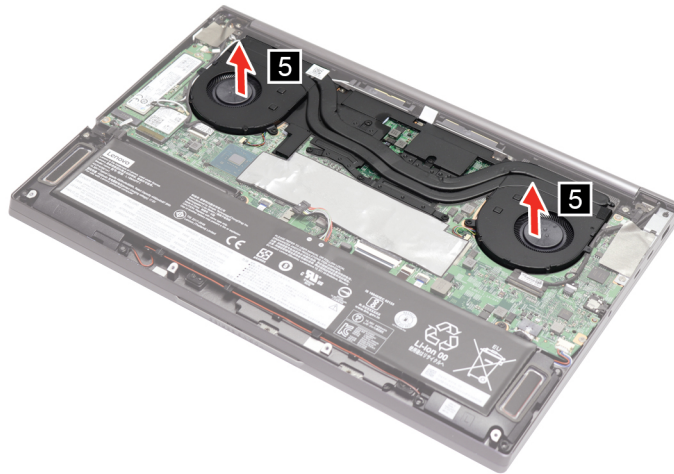
Figure 17. Remove the thermal module
