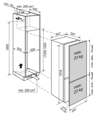
IK277BN / IK275BN Möbelfronten auf Gerätetüren verschraubt
