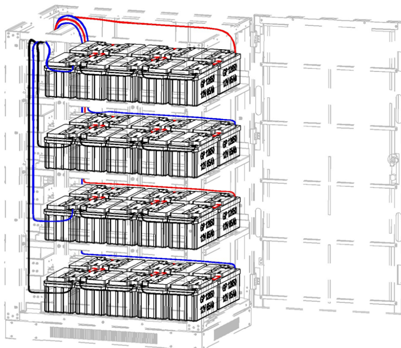
Figura 5-42: Modelo BP240V65L-NIB
