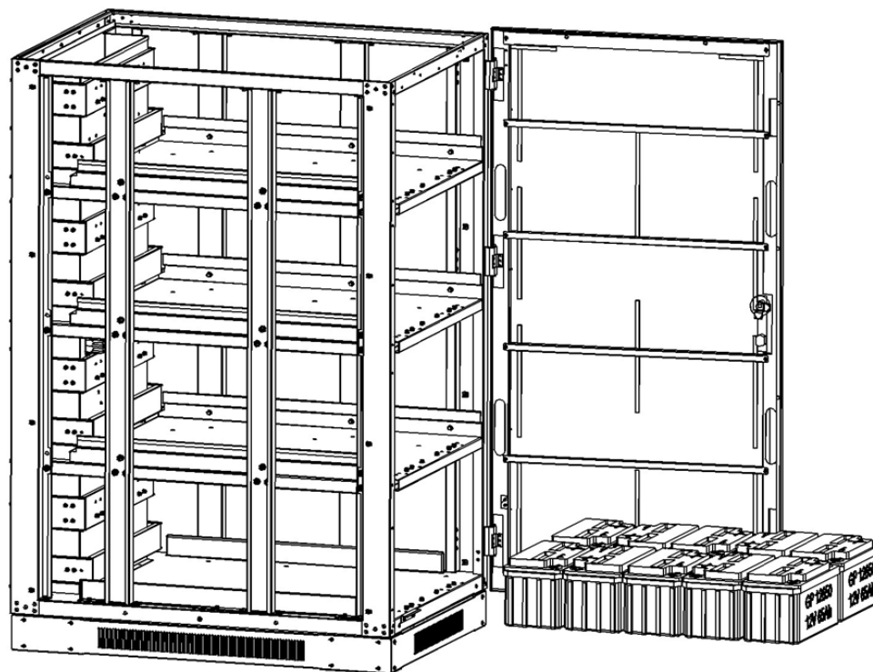
Figure 5-31 : modèle BP240V65L-NIB
