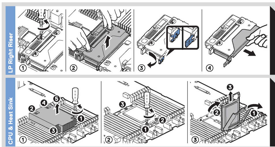
Abbildung 14. CPU und Kühlkörper und rechter Riser mit flachem Profil
