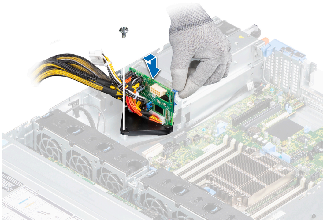
Abbildung 123. Stromzwischenplatine installieren
