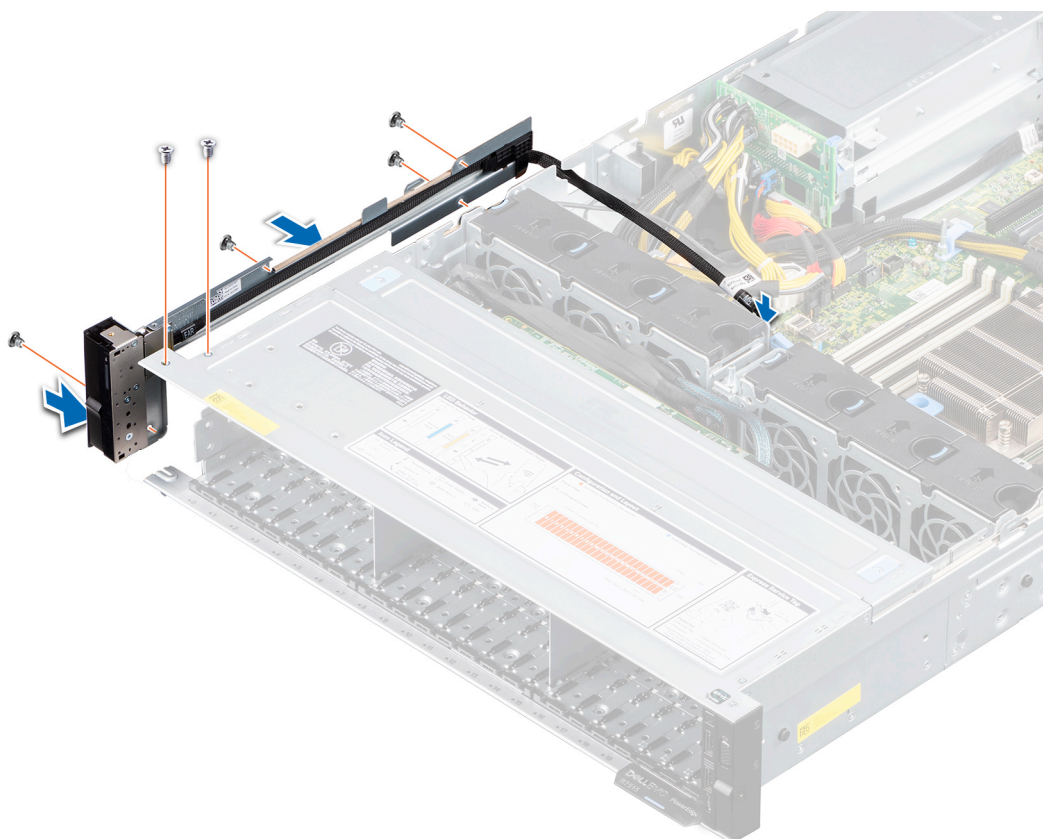
Abbildung 128. Installieren des linken Bedienfelds
