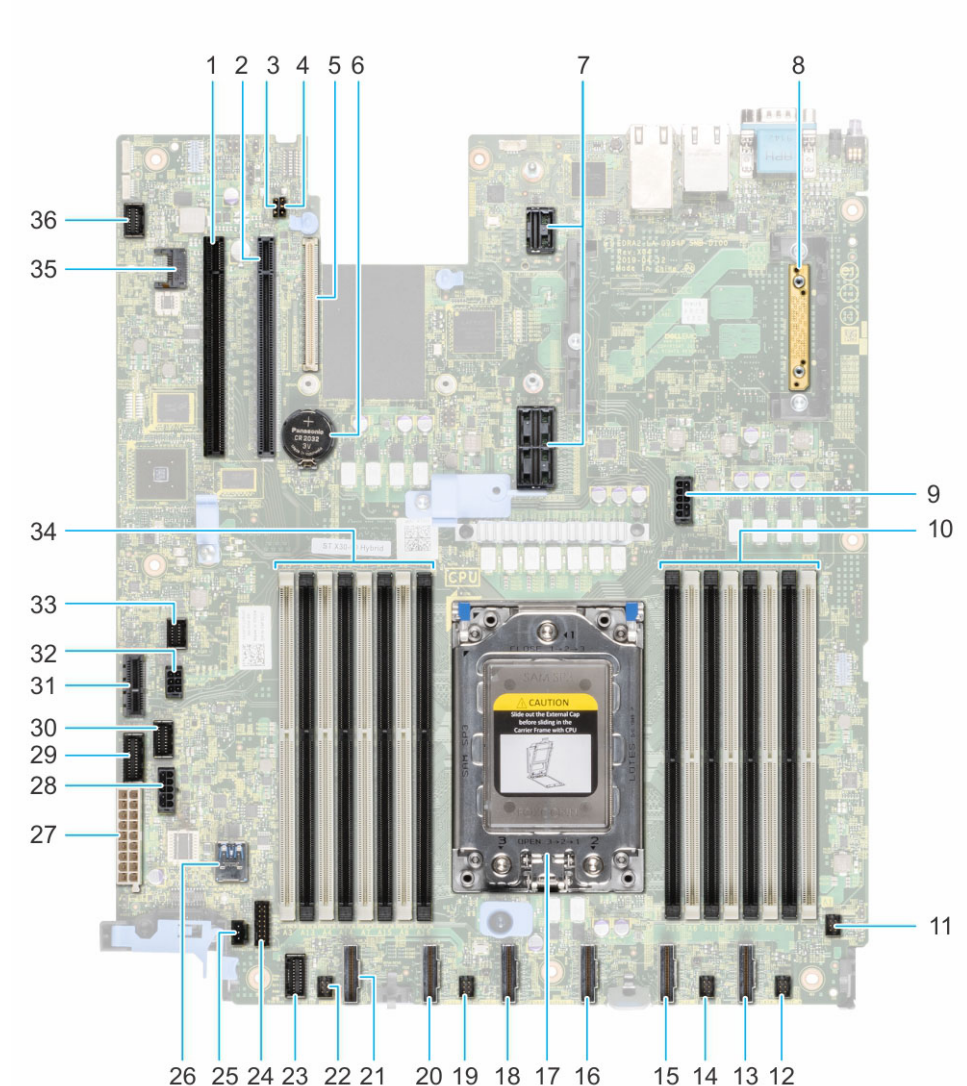
Abbildung 131. Systemplatinenanschlüsse
