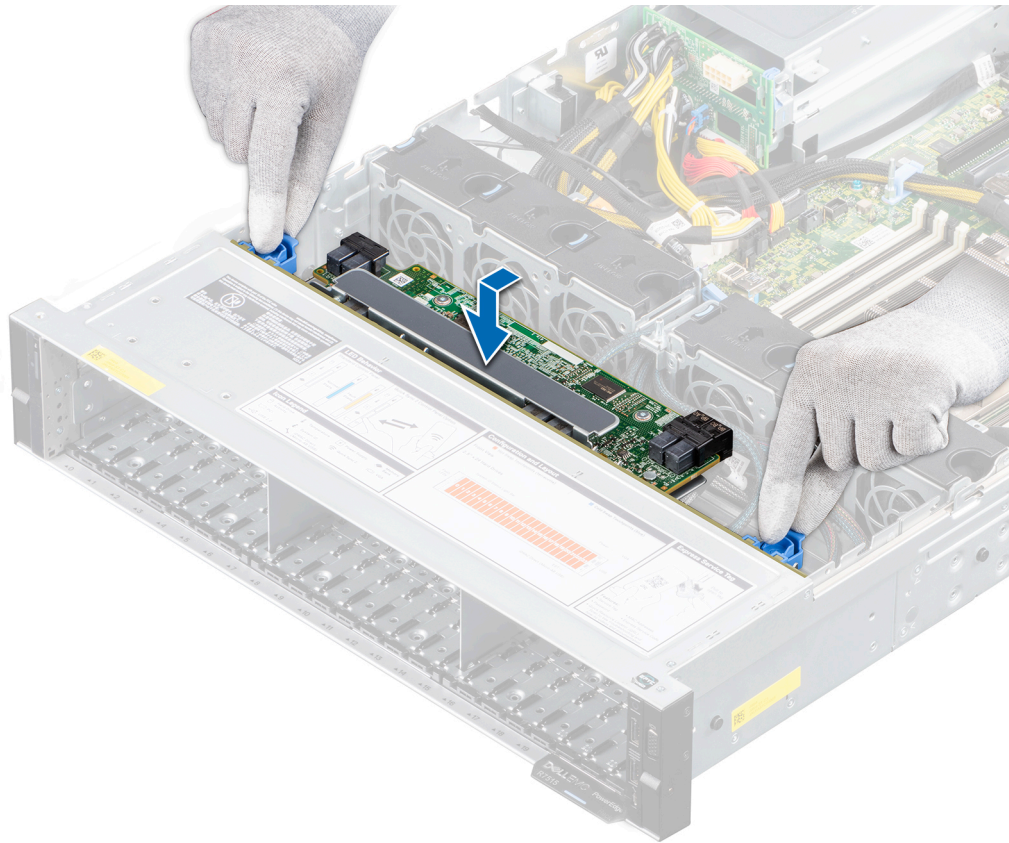
Abbildung 50. Laufwerkrückwandplatine installieren
