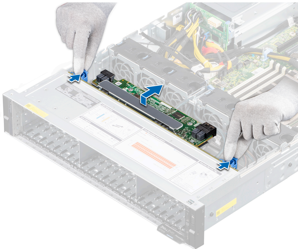
Abbildung 49. Laufwerkrückwandplatine entfernen
