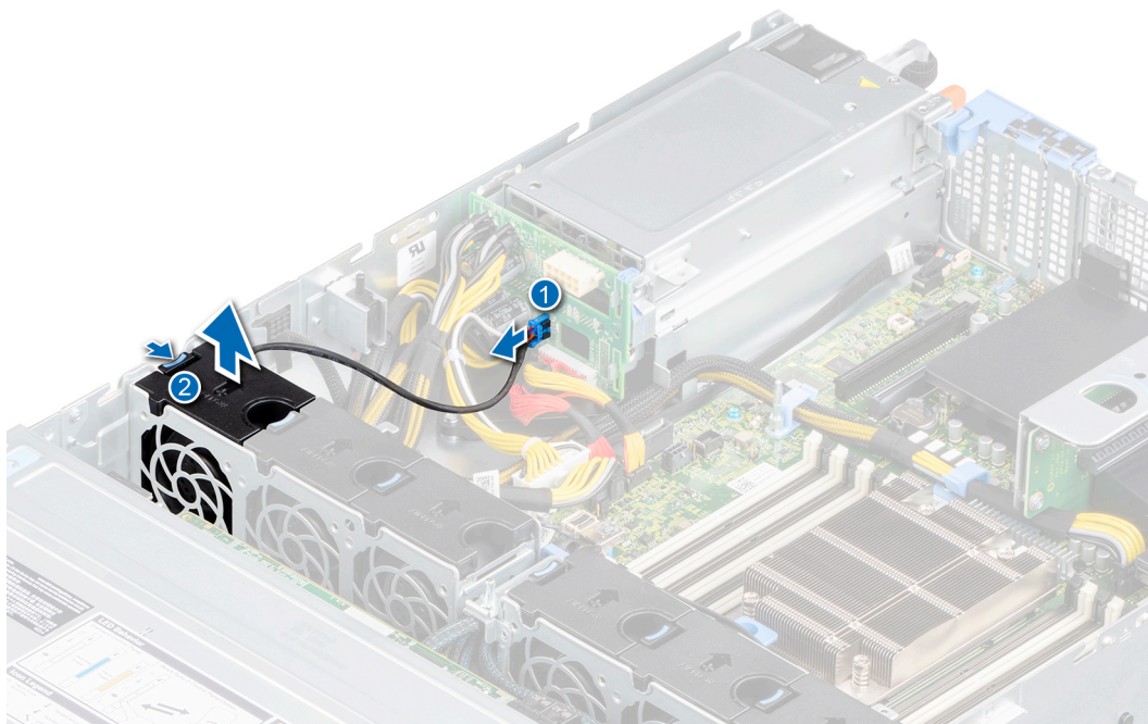
Abbildung 28. Trennen des Kabels für Lüfter 1 von der Stromzwischenplatine
