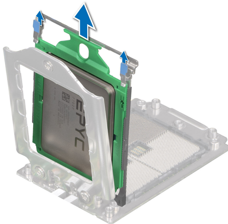
Abbildung 60. Entfernen des Prozessorträgers
