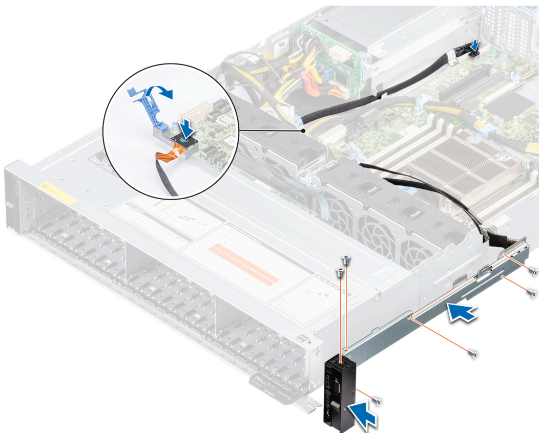
Abbildung 130. Installieren des rechten Bedienfelds
