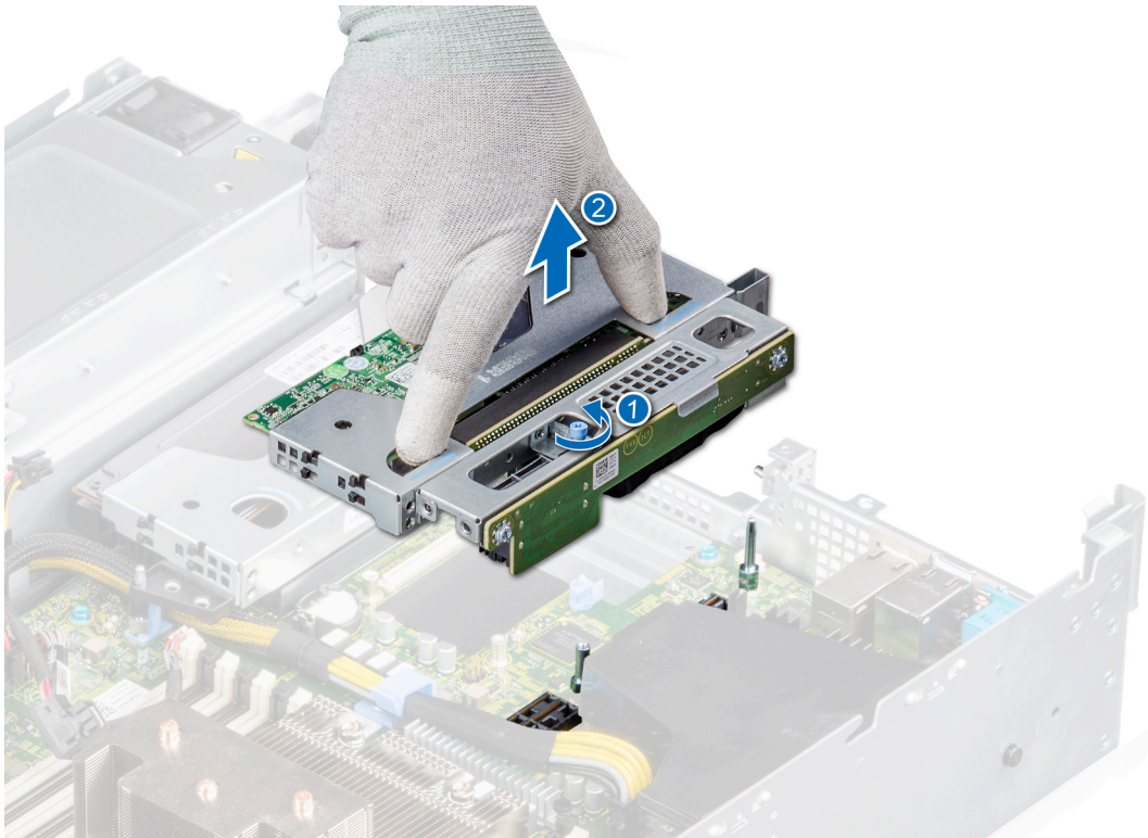
Abbildung 67. Entfernen des Riser 1A
