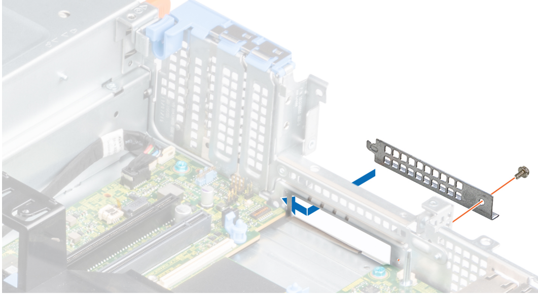
Abbildung 102. Einsetzen des Abdeckblechs für die LOM-Halterung
