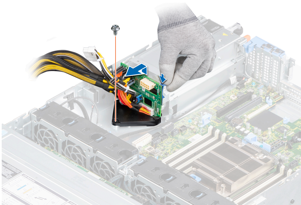
Abbildung 122. Stromzwischenplatine entfernen
