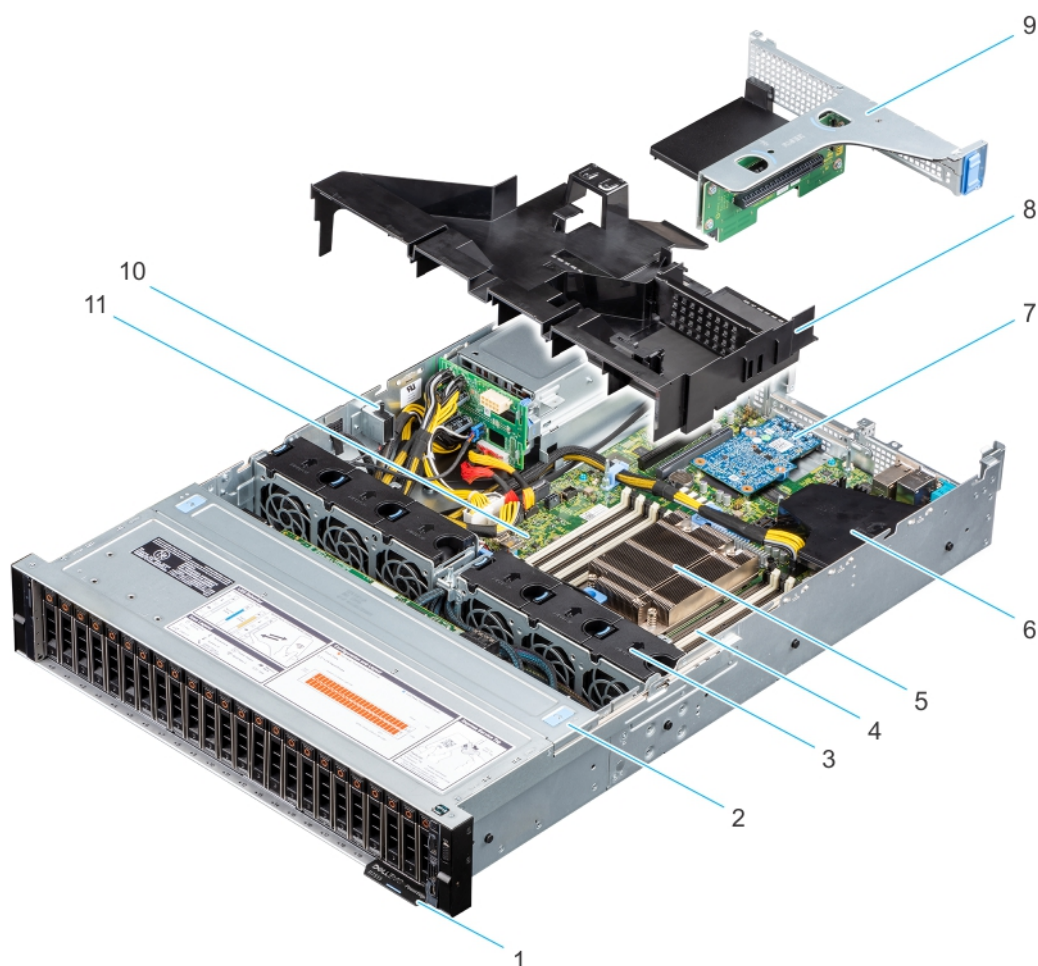
Abbildung 9. Das Systeminnere
