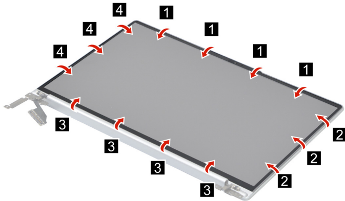
Figure 29. Remove the LCD bezel.
