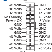
C ATX_PWR
