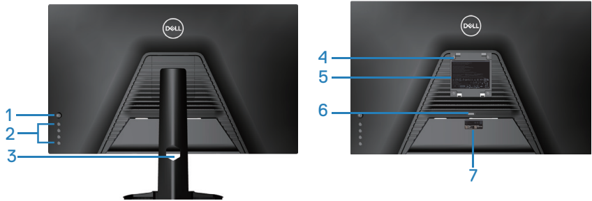
Vue de derrière avec la base du moniteur
