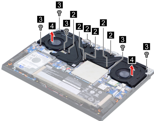
Figure 15. Remove the thermal module
