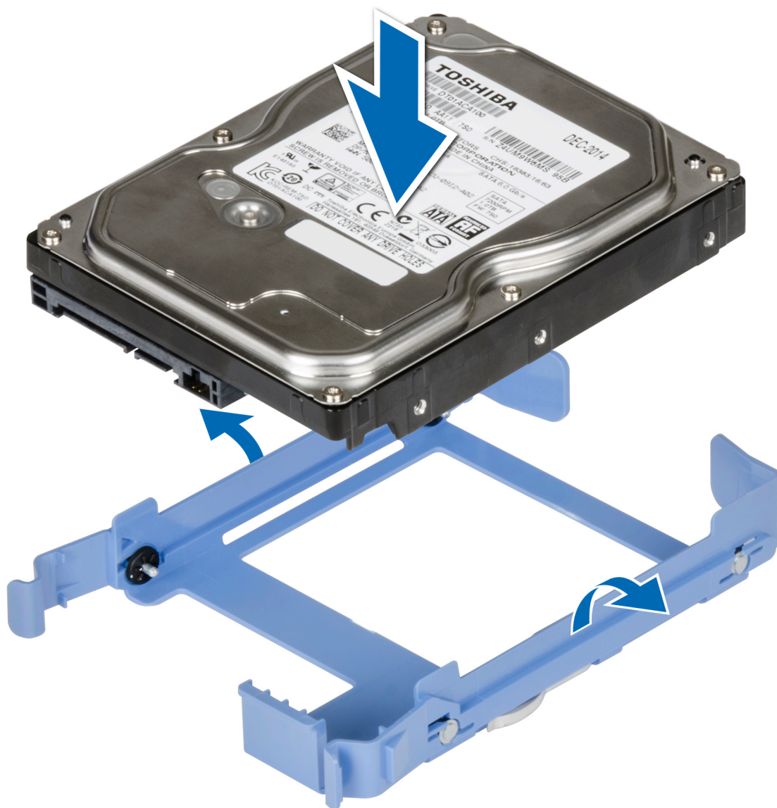
Ilustración 16. Instalación de una unidad en el portaunidades
