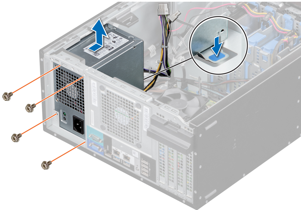
Ilustración 43. Extracción de la PSU
