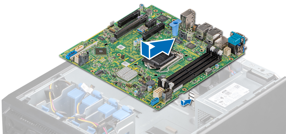
Ilustración 52. Instalación de la placa base
