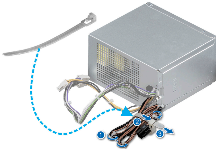
Ilustración 44. Inclusión del cable P3 de la PSU
