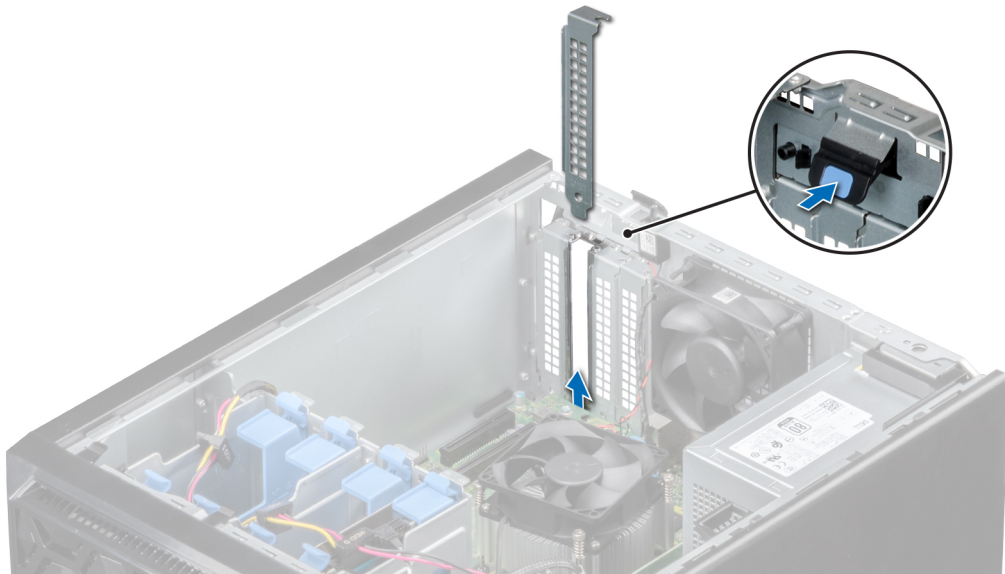
Ilustración 30. Extracción del soporte de relleno
