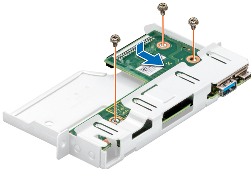
Ilustración 56. Instalación del panel de control
