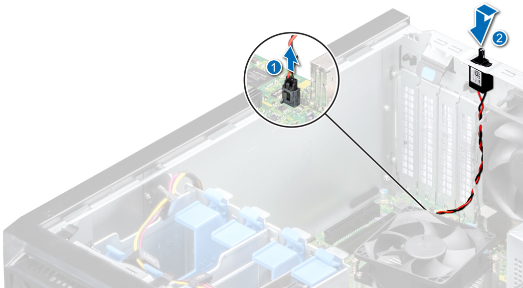
Ilustración 48. Extracción del interruptor de intrusiones
