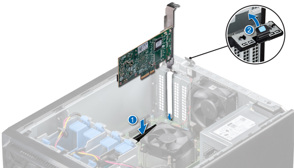
Ilustración 31. Instalación de una tarjeta de expansión de PCIe
