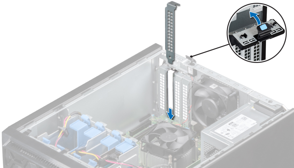
Ilustración 29. Instalación del soporte de relleno
