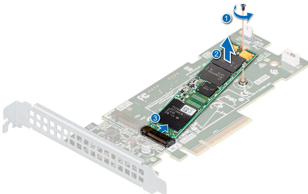
Ilustración 36. Extracción del módulo M.2 SSD
