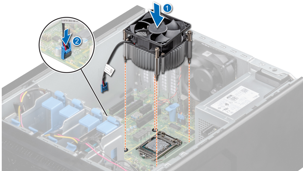
Ilustración 42. Instalación del disipador de calor
