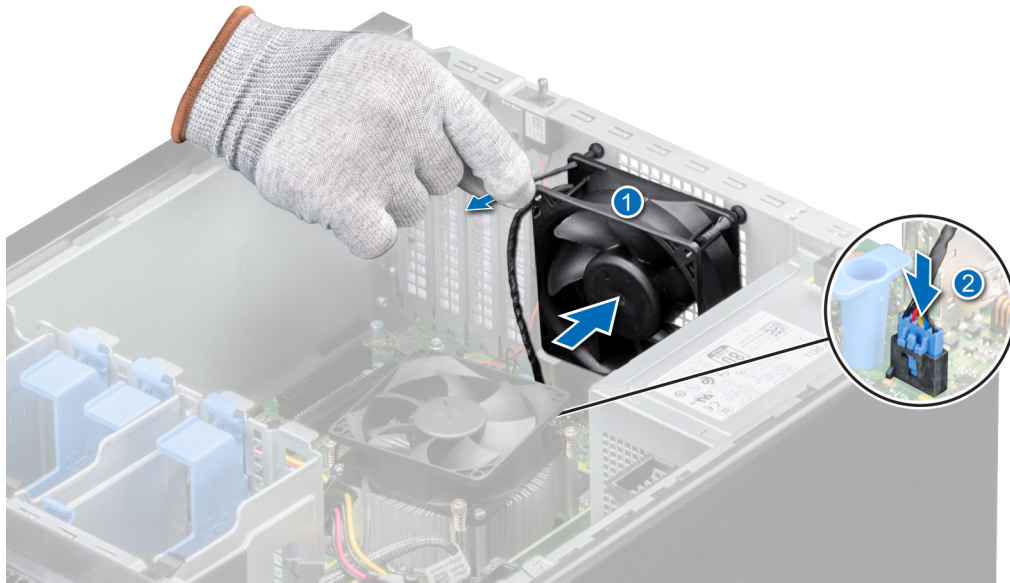
Ilustración 27. Instalación de un ventilador de refrigeración
