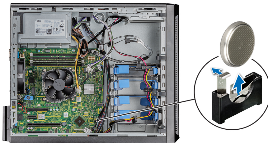
Ilustración 46. Extracción de la batería del sistema
