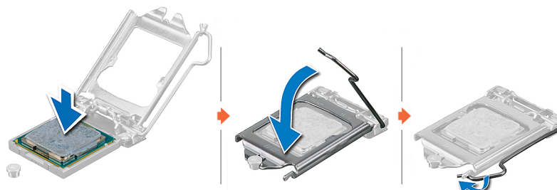
Ilustración 40. Instalación del procesador
