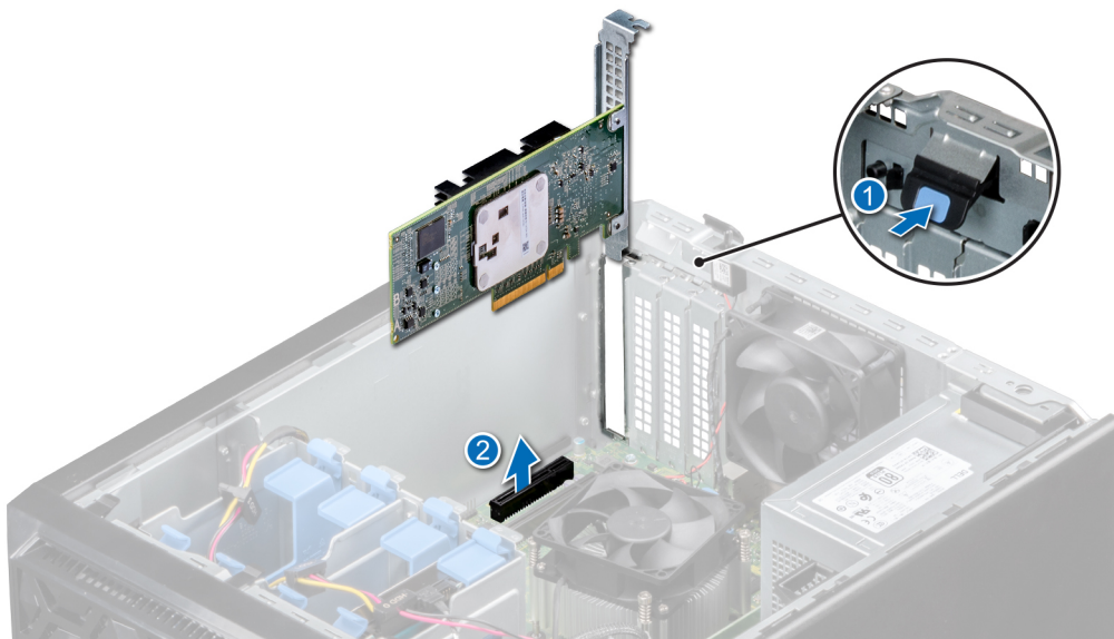
Ilustración 32. Extracción de la tarjeta controladora de almacenamiento integrada
