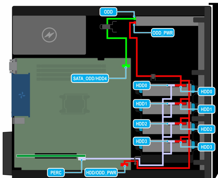
Ilustración 35. Colocación de los cables: cuatro unidades SAS cableadas de 3.5 pulgadas con tarjeta controladora de almacenamiento
