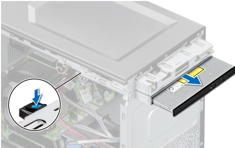
Ilustración 21. Extracción de la unidad óptica
