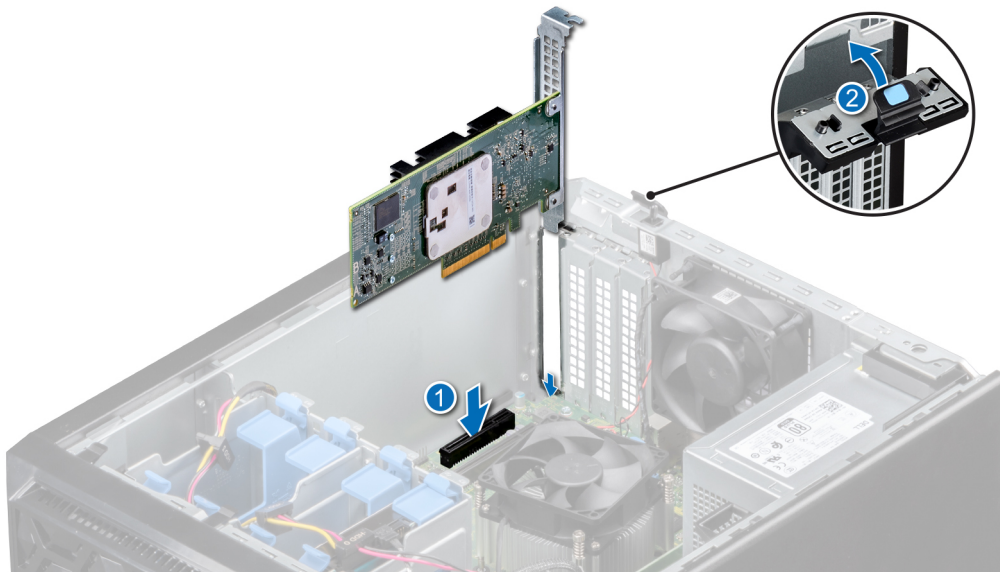
Ilustración 33. Instalación de una tarjeta integrada de la controladora de almacenamiento
