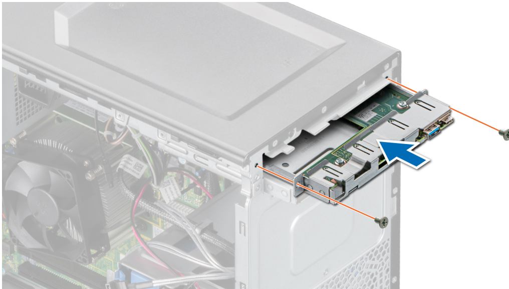
Ilustración 57. Instalación de la canastilla del panel de control
