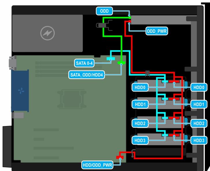
Ilustración 34. Colocación de los cables: cuatro unidades SATA cableadas de 3.5 pulgadas
