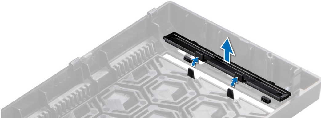
Ilustración 17. Extracción de la unidad óptica de relleno del bisel frontal
