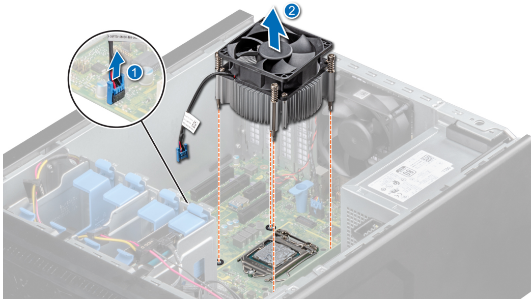
Ilustración 38. Extracción del disipador de calor
