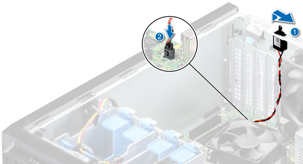
Ilustración 49. Instalación del interruptor de intrusiones
