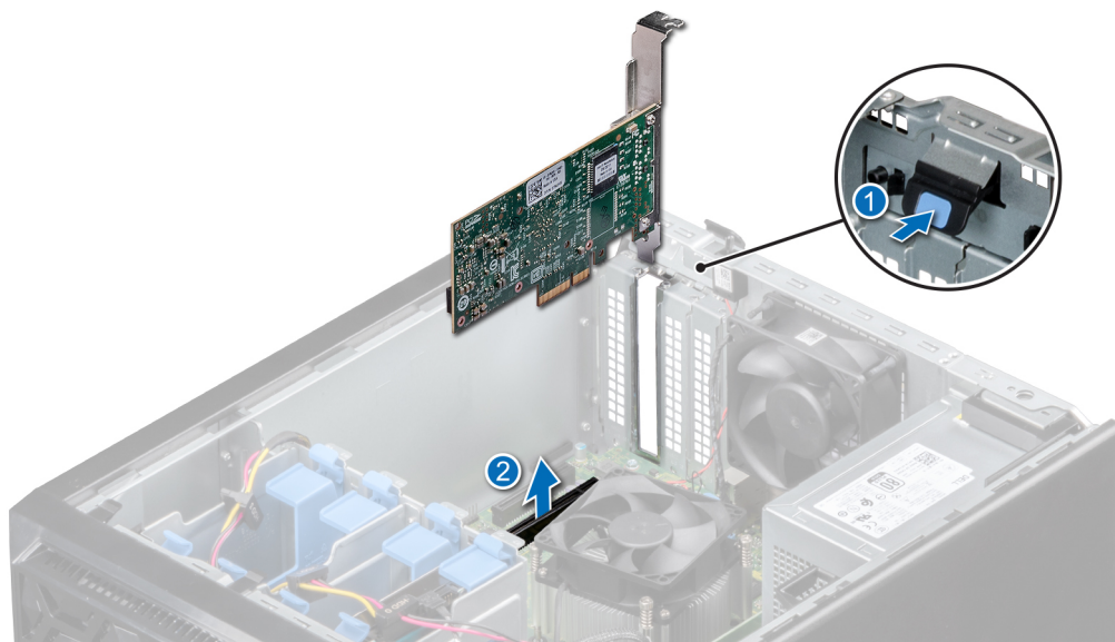
Ilustración 28. Extracción de una tarjeta de expansión de PCIe
