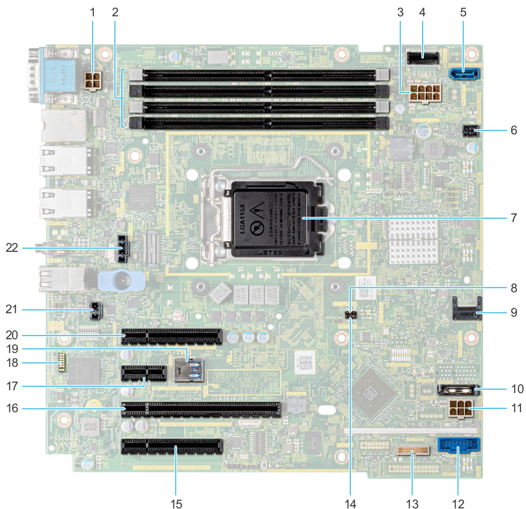
Ilustración 58. Puentes y conectores de la placa base
