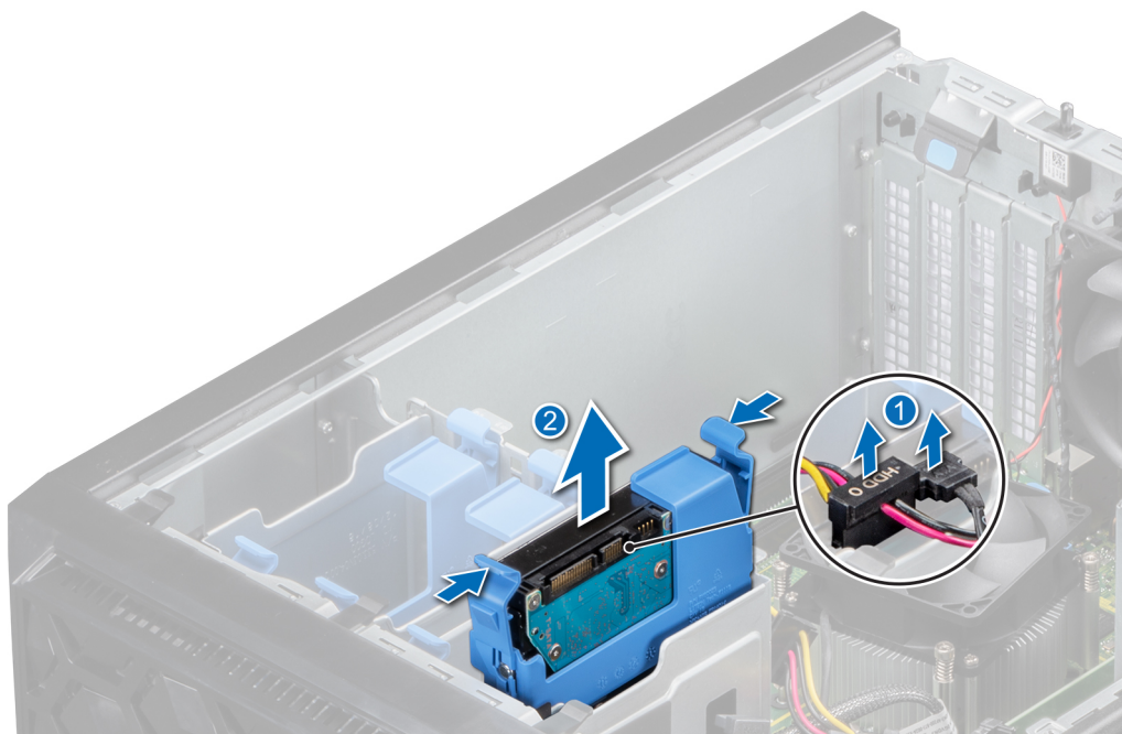
Ilustración 13. Extracción del portaunidades del compartimento para unidad
