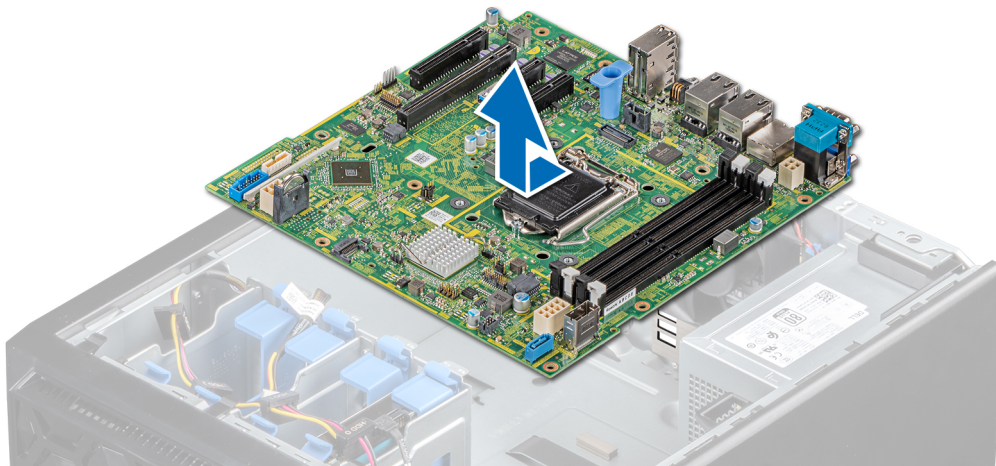
Ilustración 51. Extracción de la placa base
