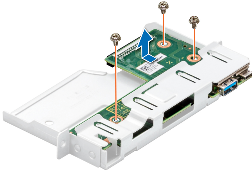
Ilustración 55. Extracción del panel de control
