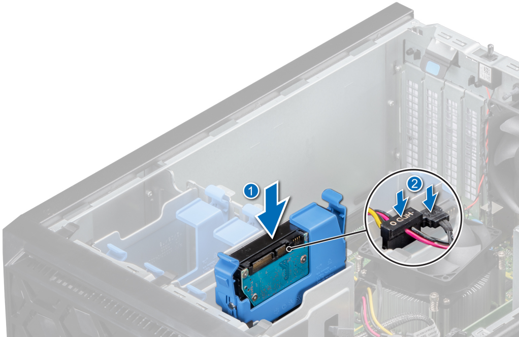
Ilustración 14. Instalación de un portaunidades en la bahía de unidades
