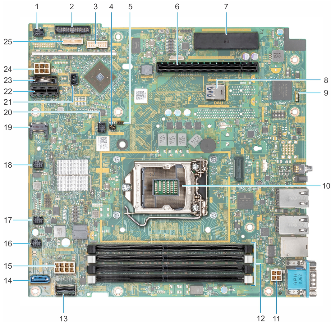
Abbildung 82. Systemplatinenanschlüsse
