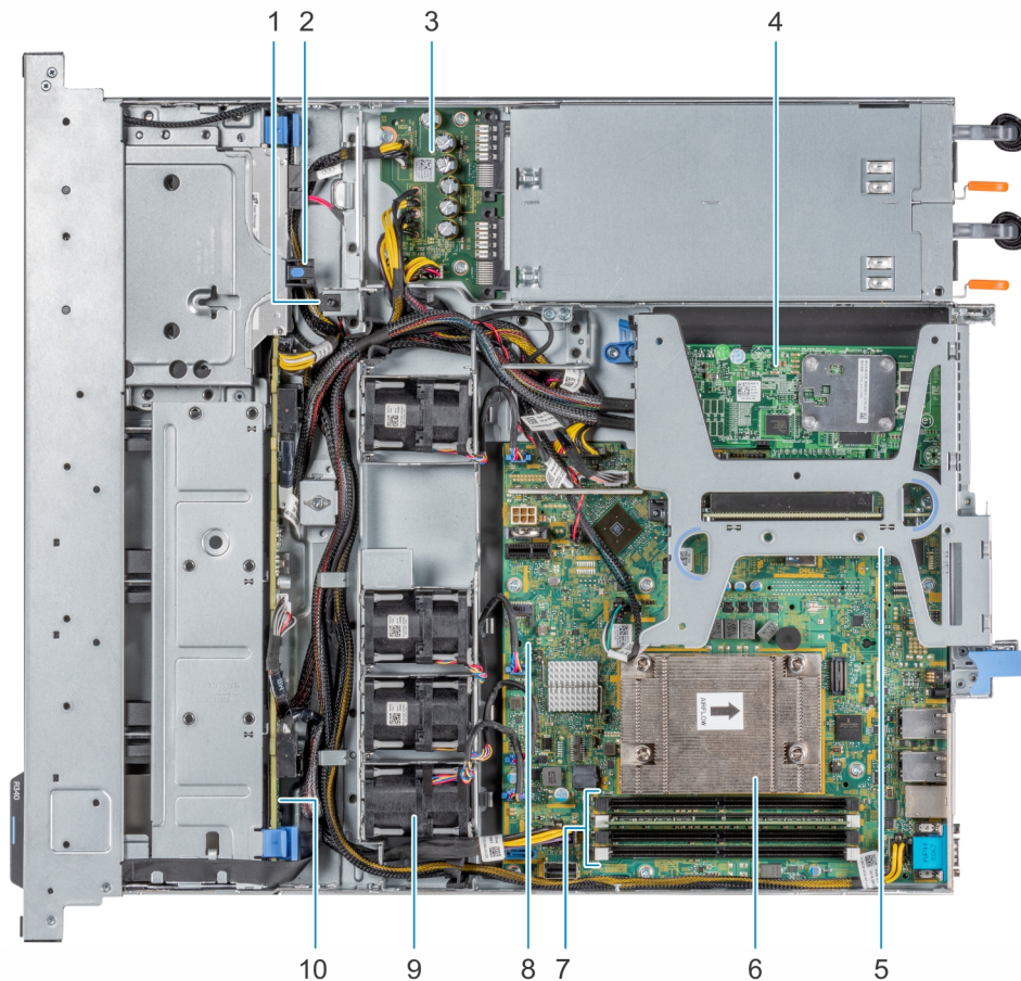
Abbildung 6. Das Systeminnere
