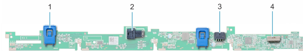
Abbildung 62. 3,5-Zoll-SAS/SATA-Rückwandplatine (x4)
