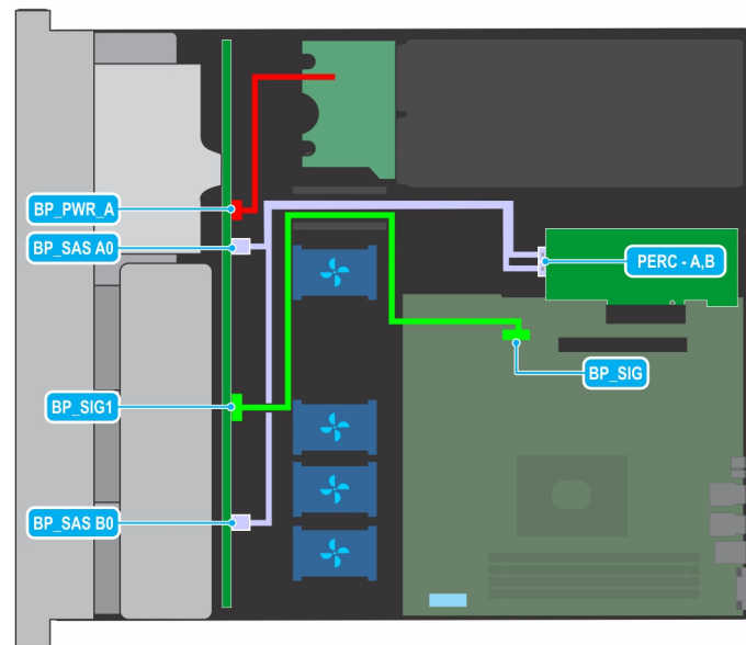
Abbildung 66. Kabelführung – 8 x 2,5-Zoll-SAS-Rückwandplatine mit PERC
