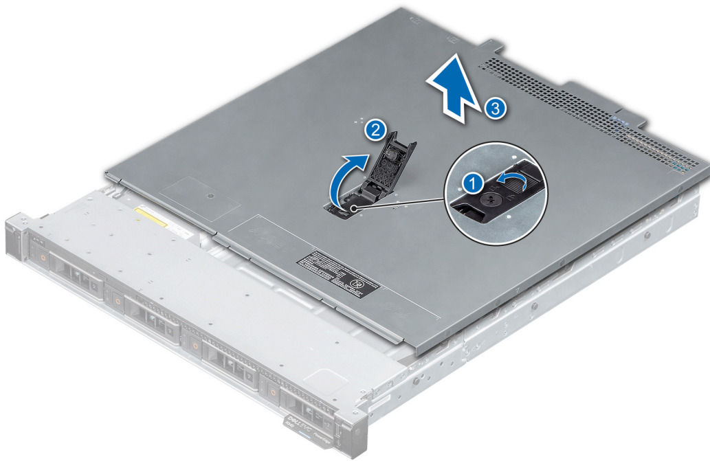
Abbildung 15. Systemabdeckung entfernen
