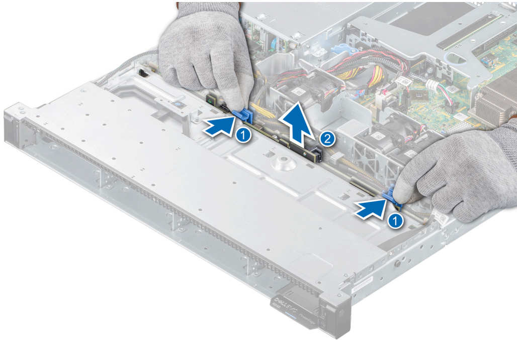
Abbildung 63. Laufwerkrückwandplatine entfernen
