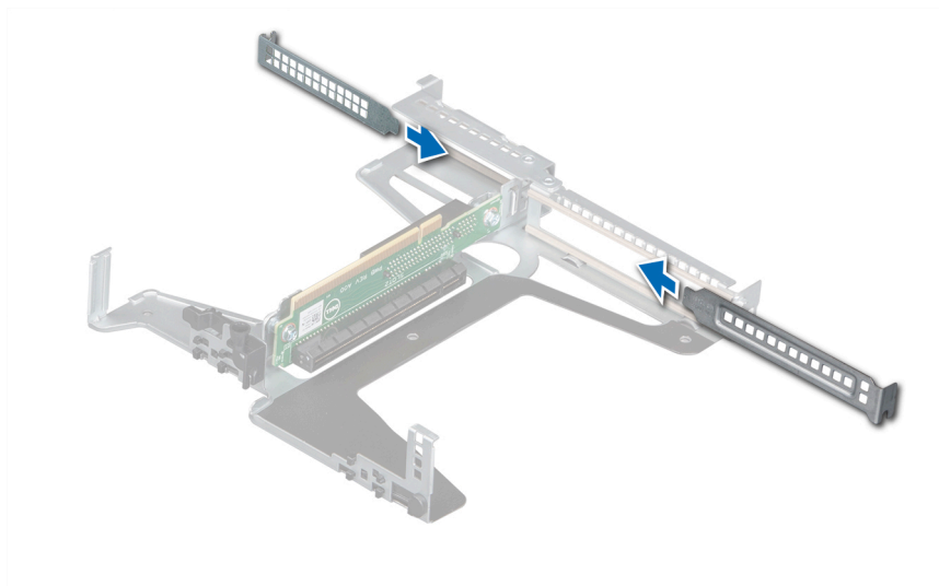
Abbildung 42. Installieren des Abdeckblechs der Erweiterungskarte
