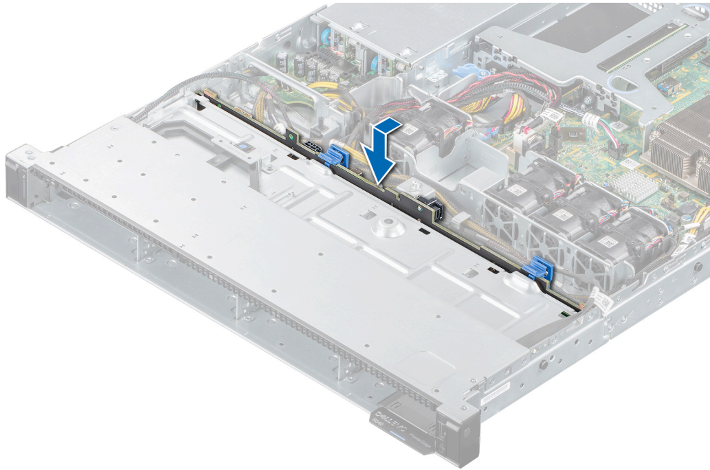
Abbildung 64. Laufwerkrückwandplatine installieren
