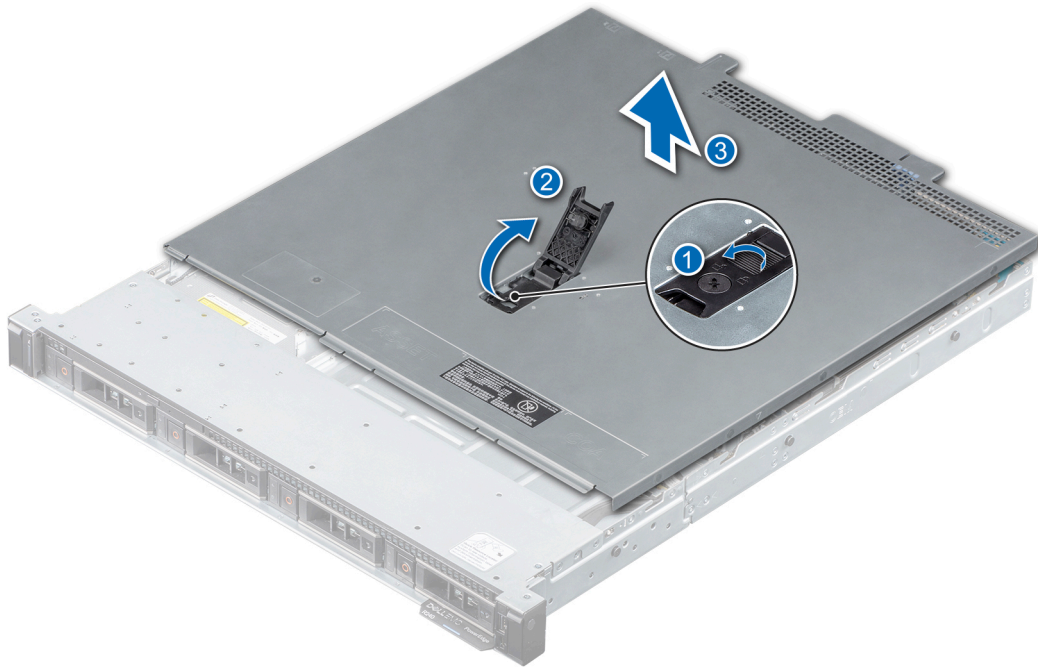
Ilustración 11. Extracción de la cubierta del sistema
