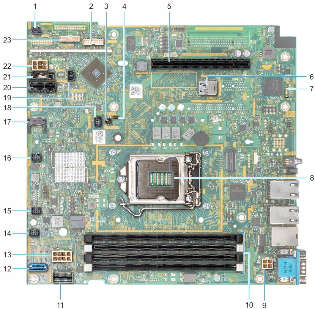
Ilustración 79. Conectores de la placa base
