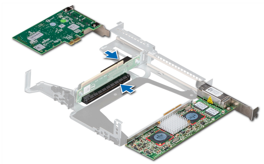
Ilustración 46. Instalación de una tarjeta de expansión en el soporte vertical para tarjetas de expansión
