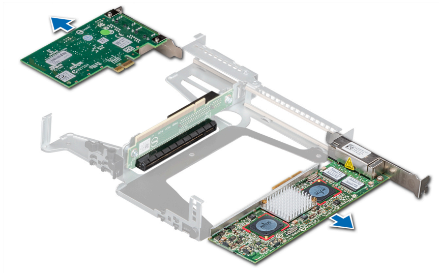
Ilustración 43. Extracción de una tarjeta de expansión del soporte vertical para tarjetas de expansión
