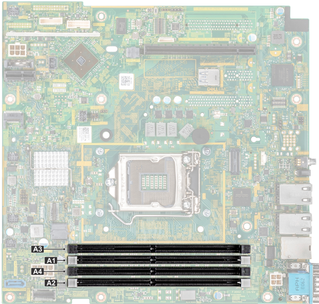
Ilustración 35. Ubicaciones de los sockets de memoria
