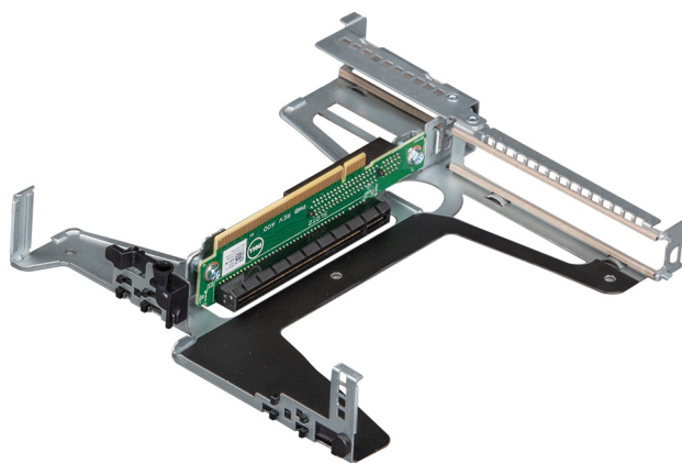
Ilustración 38. Soporte vertical para tarjetas de expansión
