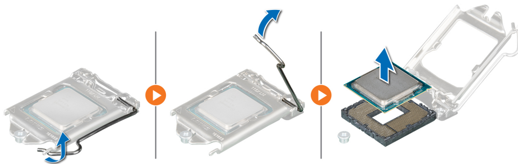
Ilustración 54. Extracción del procesador
