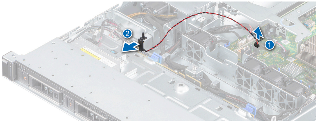
Ilustración 33. Extracción del interruptor de intrusiones
