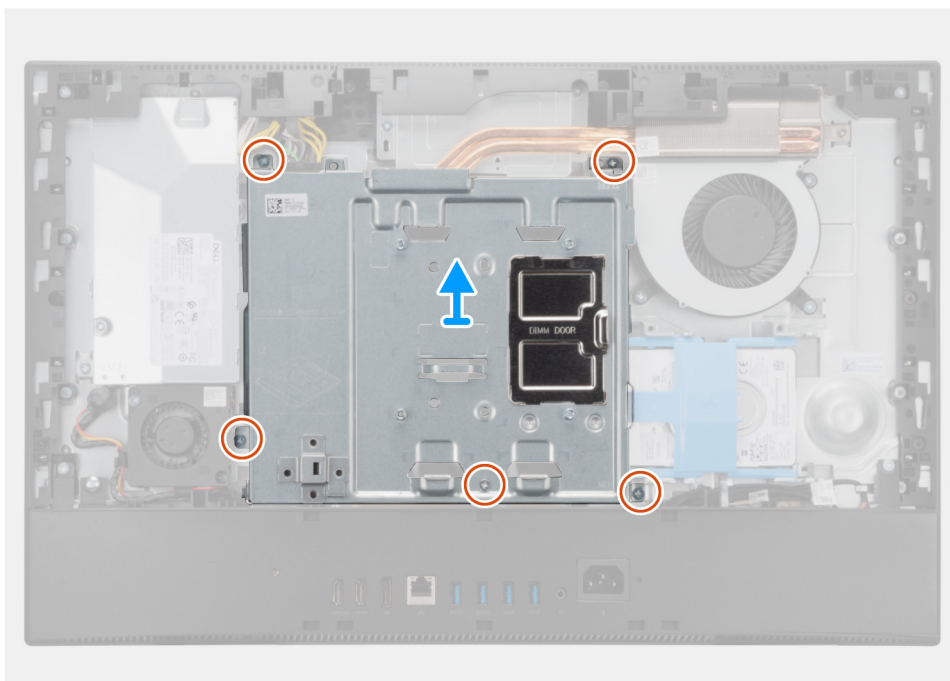
5x M3x5
