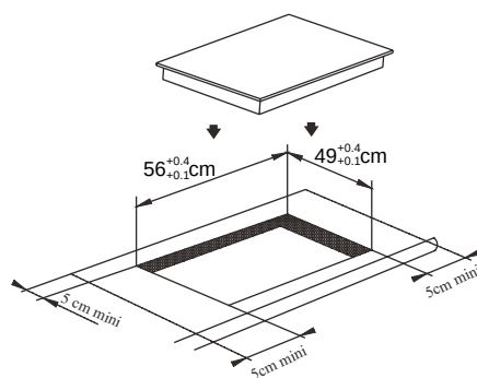
(tesnilo) Slika 1
