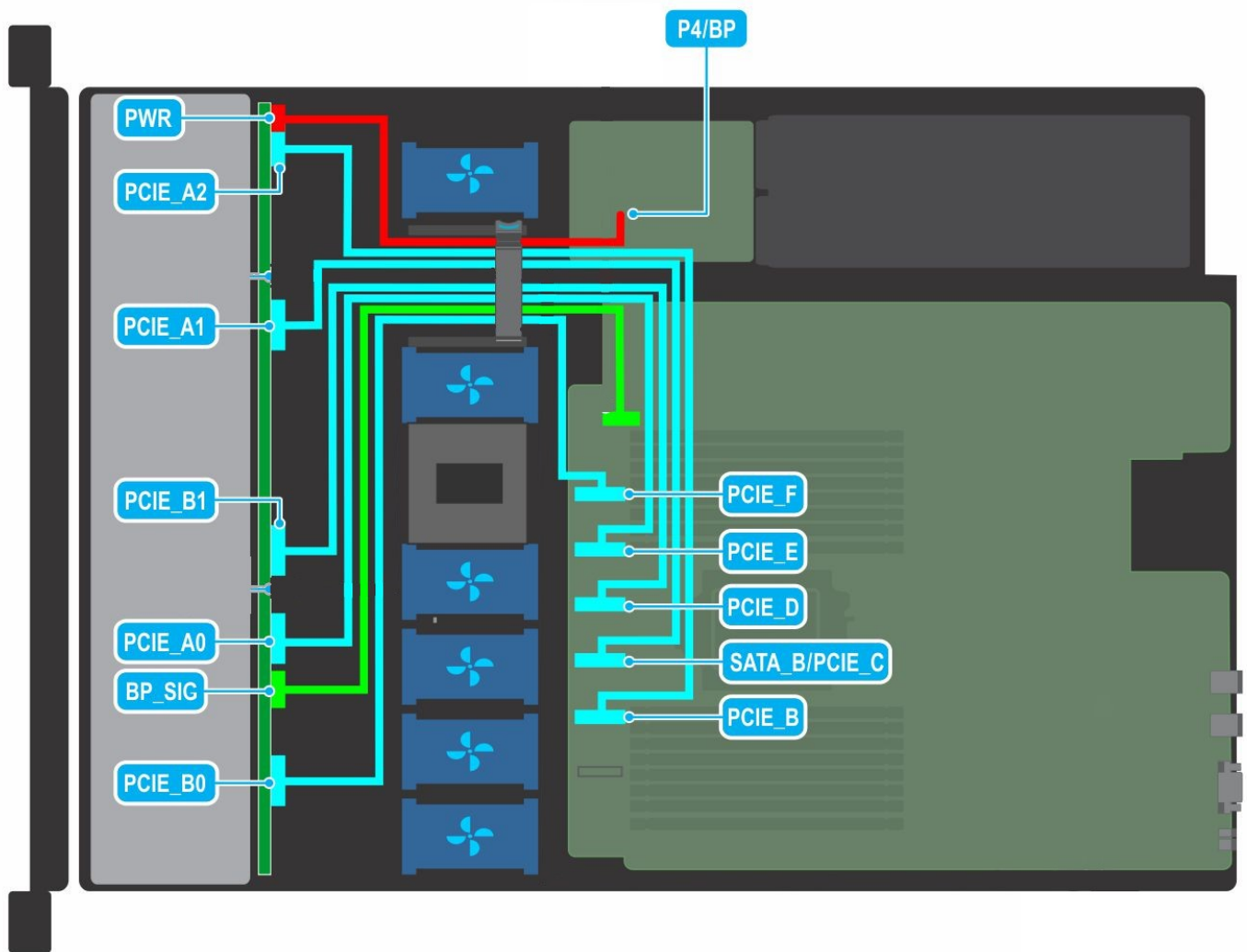
Abbildung 2. Kabelführung – 10 x 2,5-Zoll-NVMe-Laufwerksrückwandplatine
