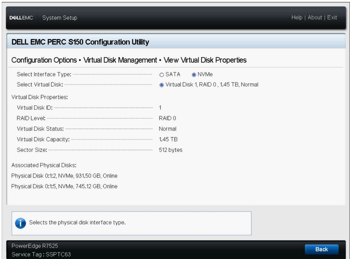
Abbildung 5. Bildschirm für Eigenschaften physischer Laufwerke
