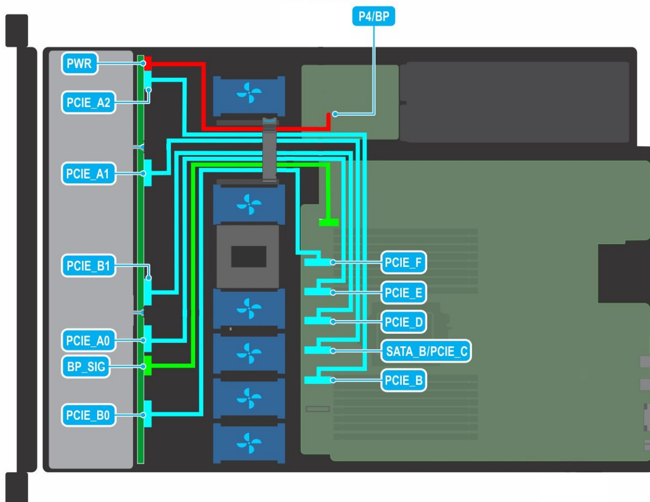
Figure 2. Acheminement des câbles – Backplane de 10 disques SATA 2,5 pouces
