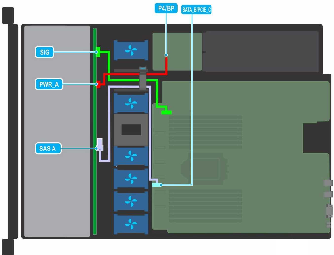
Figure 1. Acheminement des câbles – Backplane de 4 disques SATA 3,5 pouces
