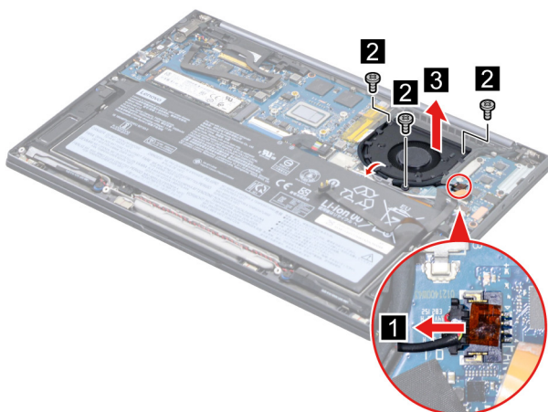
Figure 18. Remove the fan
