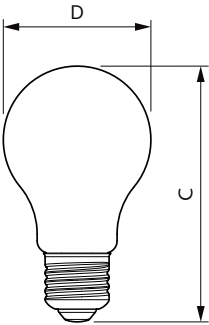
EELD Bulb A60 40W 470lm 2700K E27 D FR
