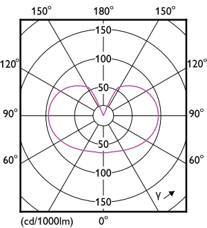
LEDbulb 8,5W E27 A60 FR
