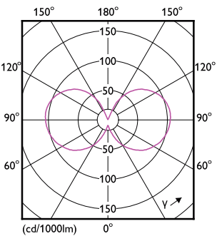
LEDbulb 6,5-60W E14 B35
