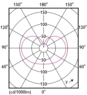
LEDbulb CLA A60 E27 806lm FR
