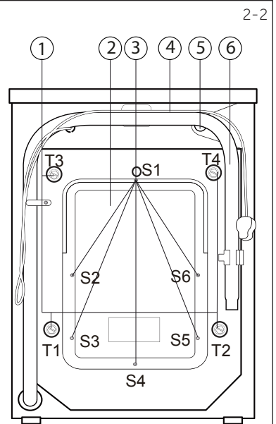
Côté arrière (Fig. 2-2) :
