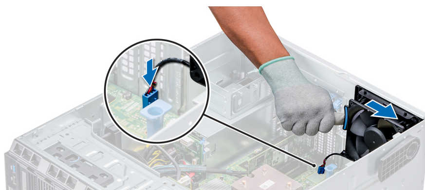
Figure 56. Installation du ventilateur de refroidissement interne
