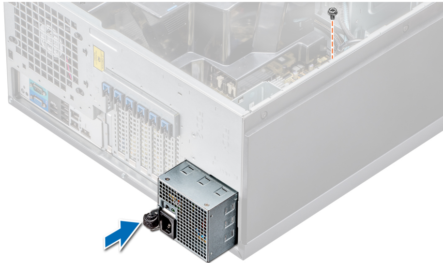
Figure 83. Installation d'un bloc d'alimentation câblé
