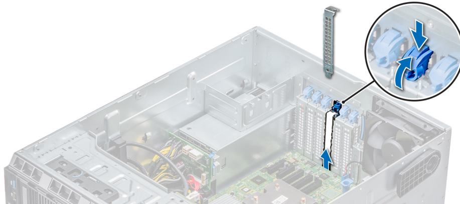
Figure 63. Retrait de la plaque de recouvrement
