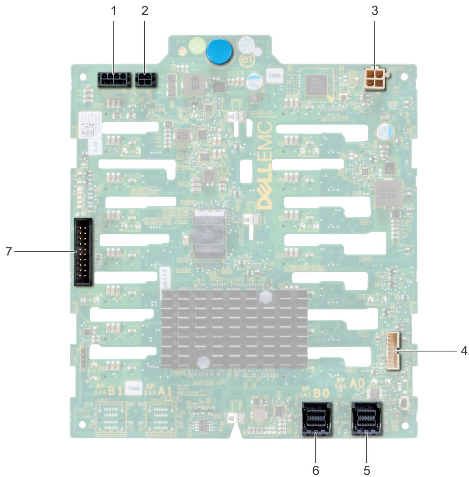
Figure 46. Fond de panier de disque x16
