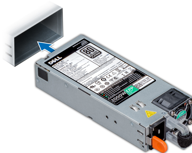
Figure 81. Installation d'une unité d'alimentation
