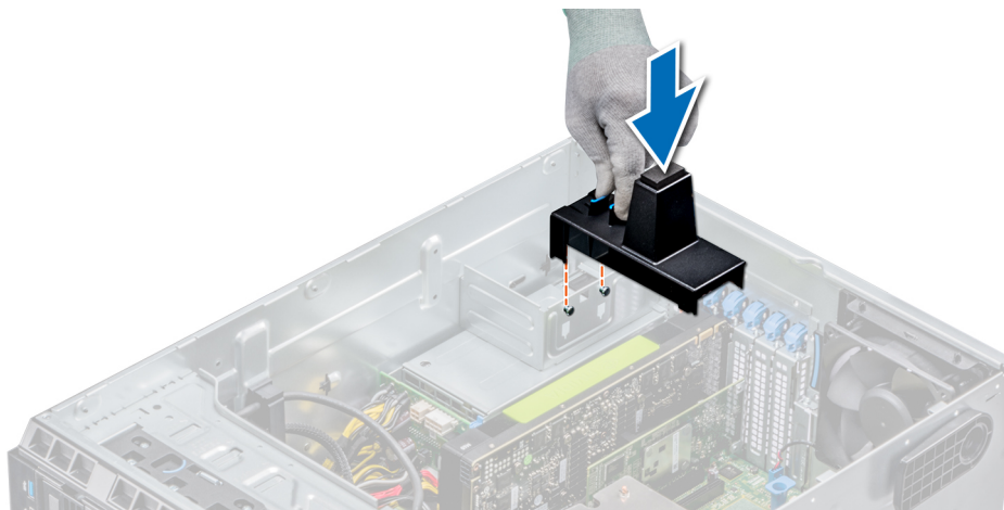
Figure 60. Installation du support de carte d'extension
