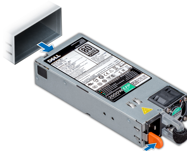
Figure 80. Retrait d'une unité d'alimentation
