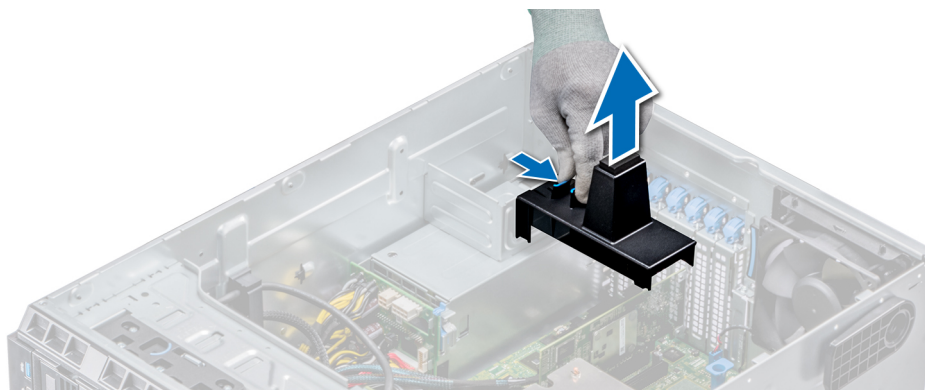
Figure 59. Retrait du support de carte d'extension
