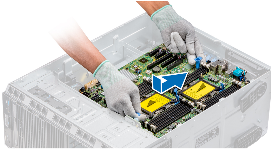
Figure 93. Installation de la carte système
