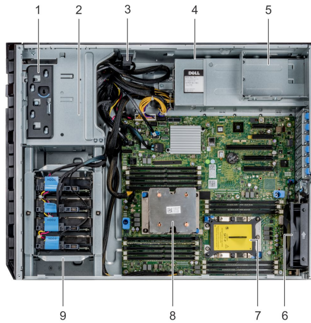
Figure 19. À l'intérieur du système - Système à disque câblé
