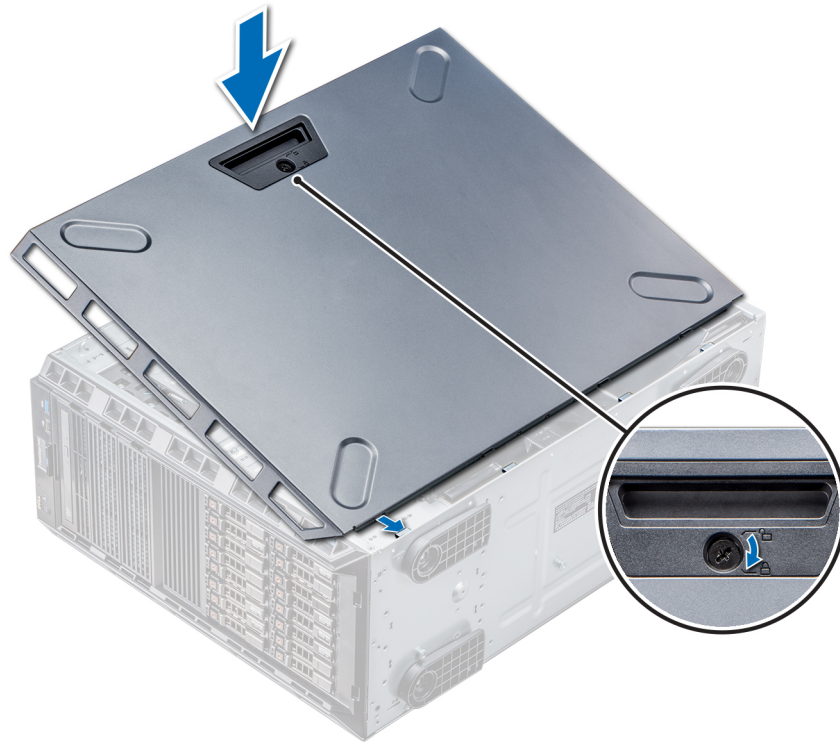
Figure 24. Installation du capot du système
