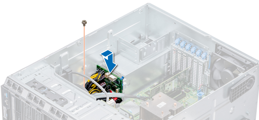
Figure 85. Installation de la carte intercalaire d'alimentation
