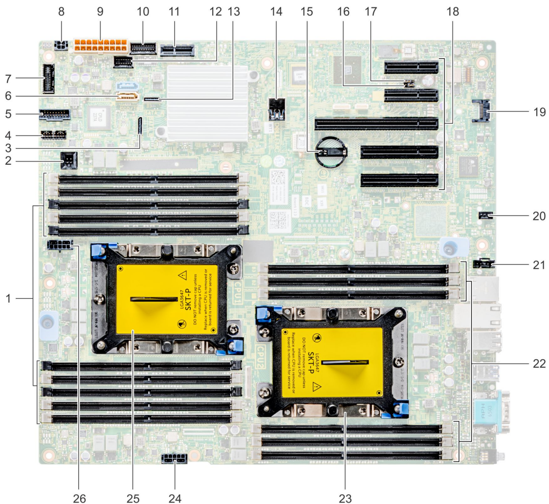
Figure 96. Connecteurs et cavaliers de la carte système du modèle T440
