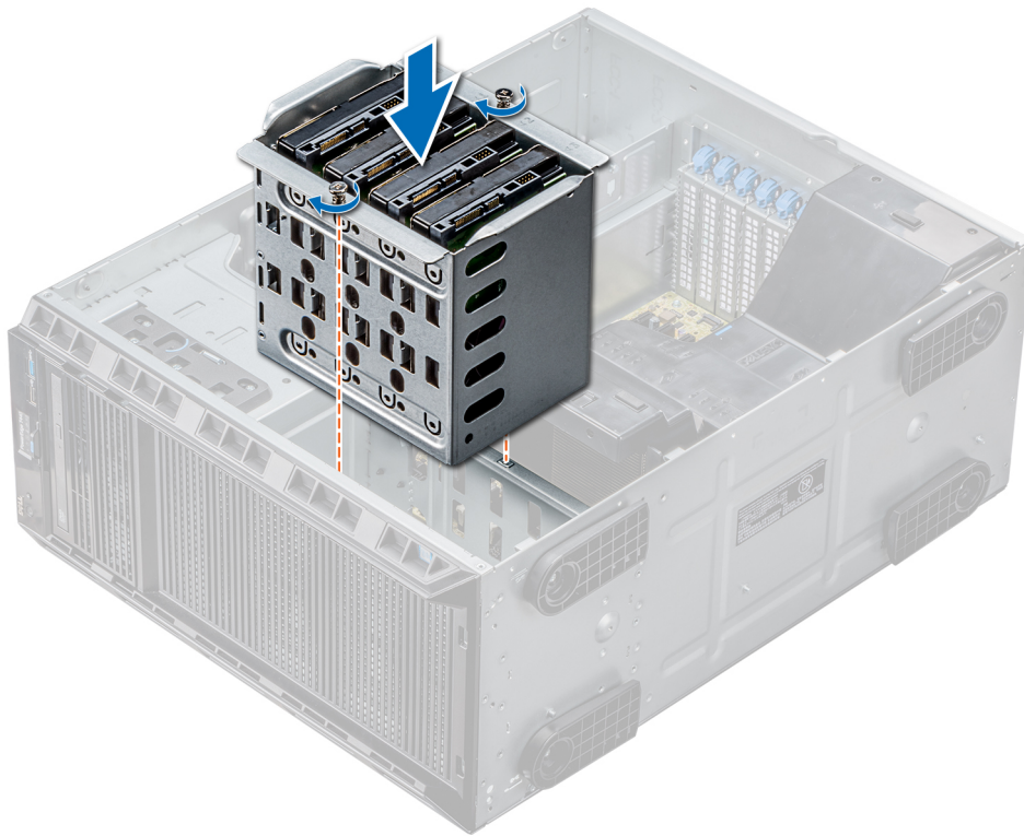
Figure 42. Installation de la baie de disque dur interne
