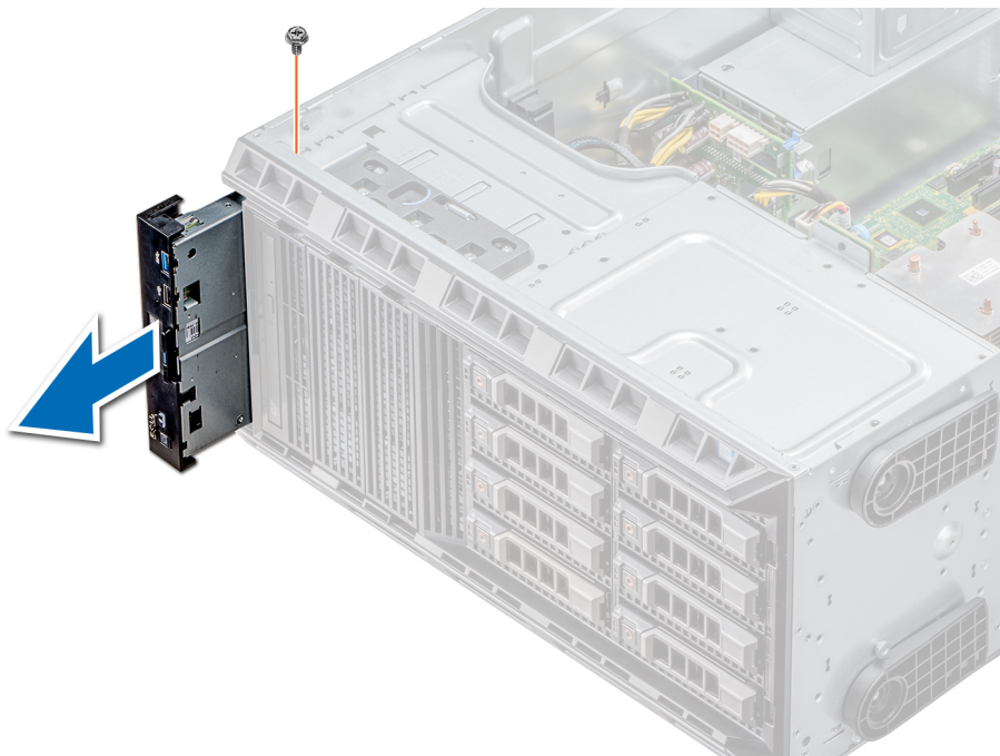
Figure 88. Retrait de l'assemblage du panneau de commande
