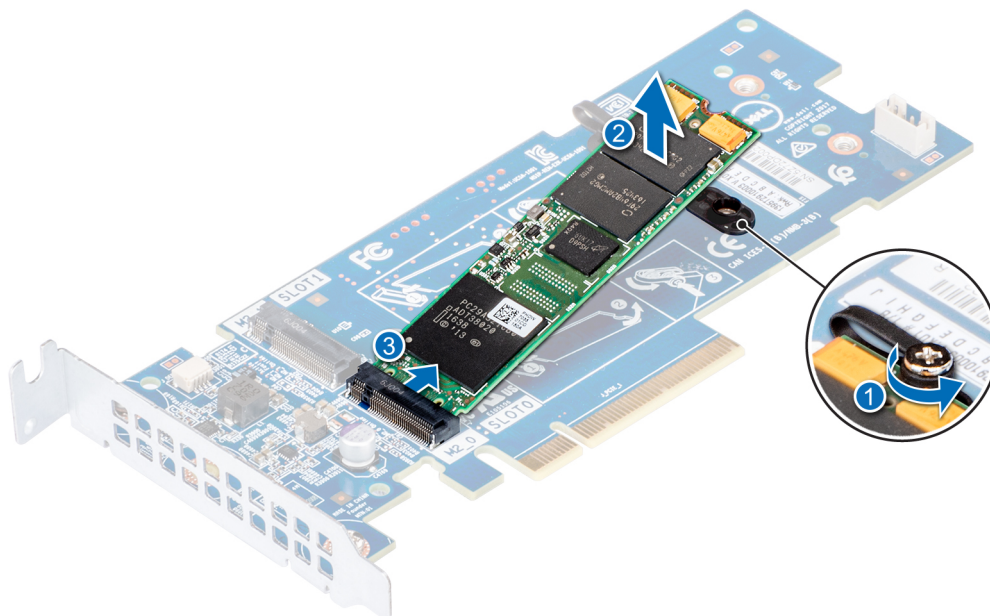
Figure 65. Retrait du module SSD M.2
