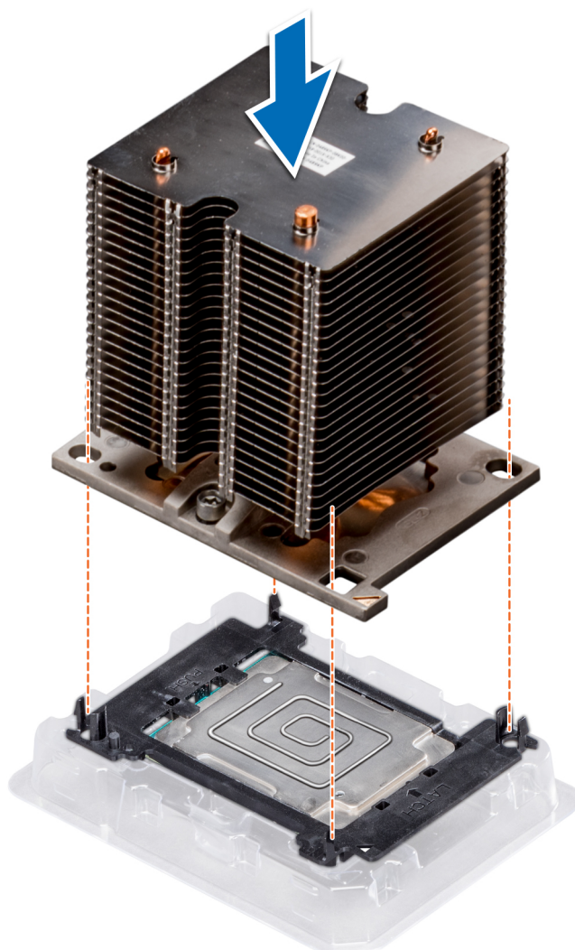
Figure 76. Installation du dissipateur de chaleur sur le processeur
