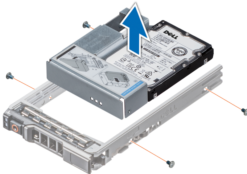
Figure 35. Retrait d'un adaptateur de disque dur de 3,5 pouces d'un support de disque dur de 3,5 pouces
