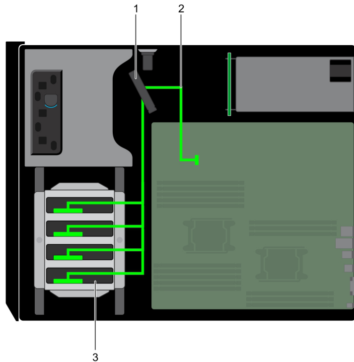
Figure 49. Acheminement des câbles : 4 disques durs câblés de 3,5 pouces
