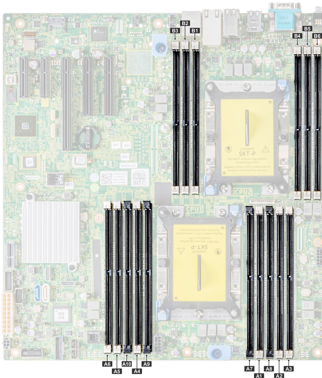
Figure 52. Vue de la mémoire système
