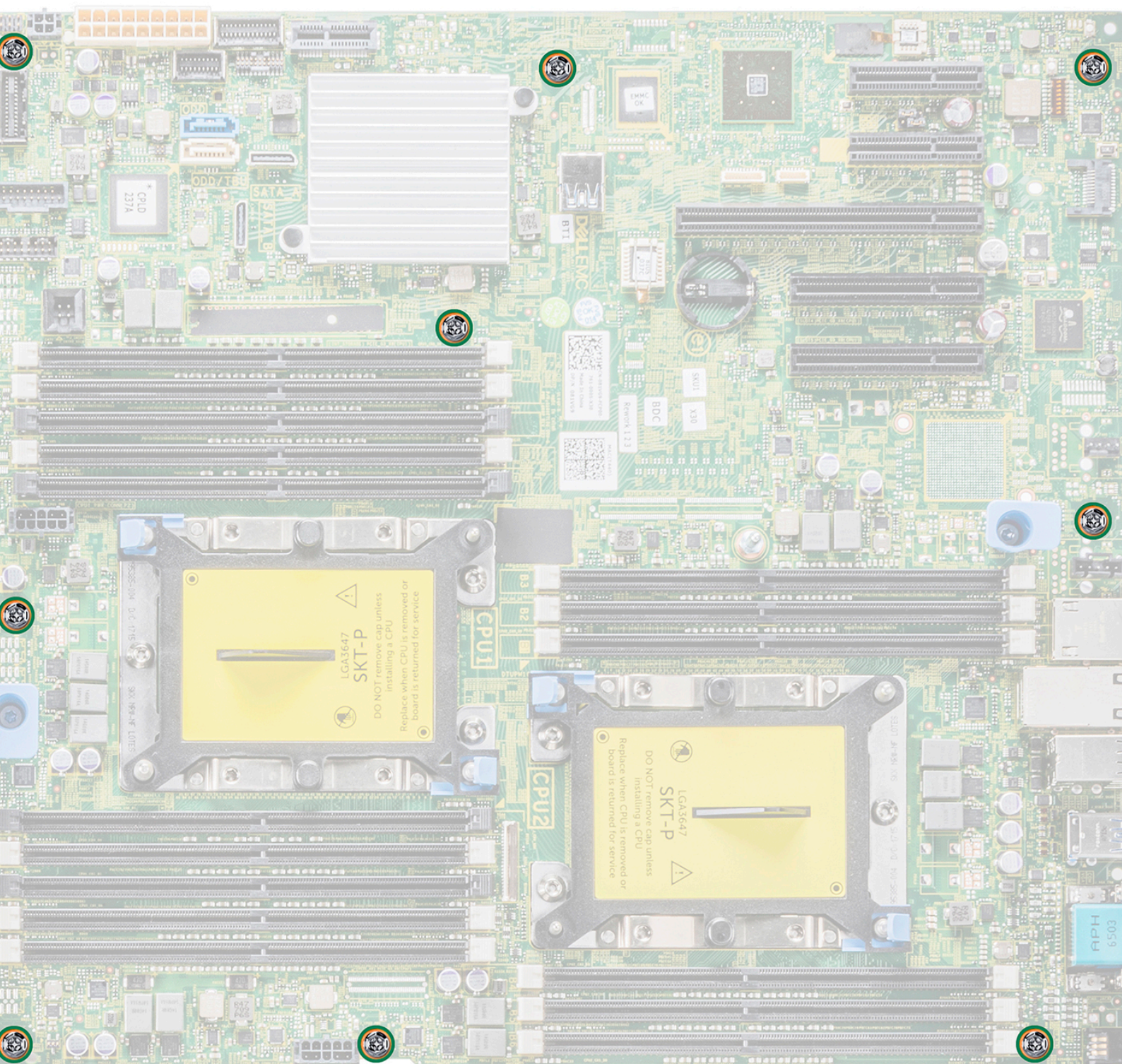
Figure 91. Vis de la carte système
