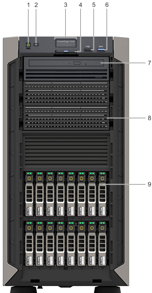
Figure 5. Vue du panneau avant d'un système à 16 disques de 2,5 pouces échangeables à chaud
