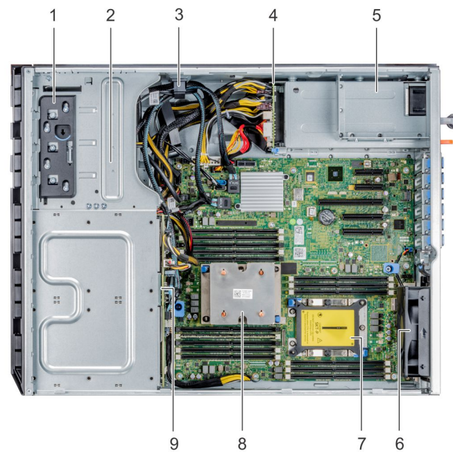
Figure 20. À l'intérieur du système - Système de disques remplaçables à chaud
