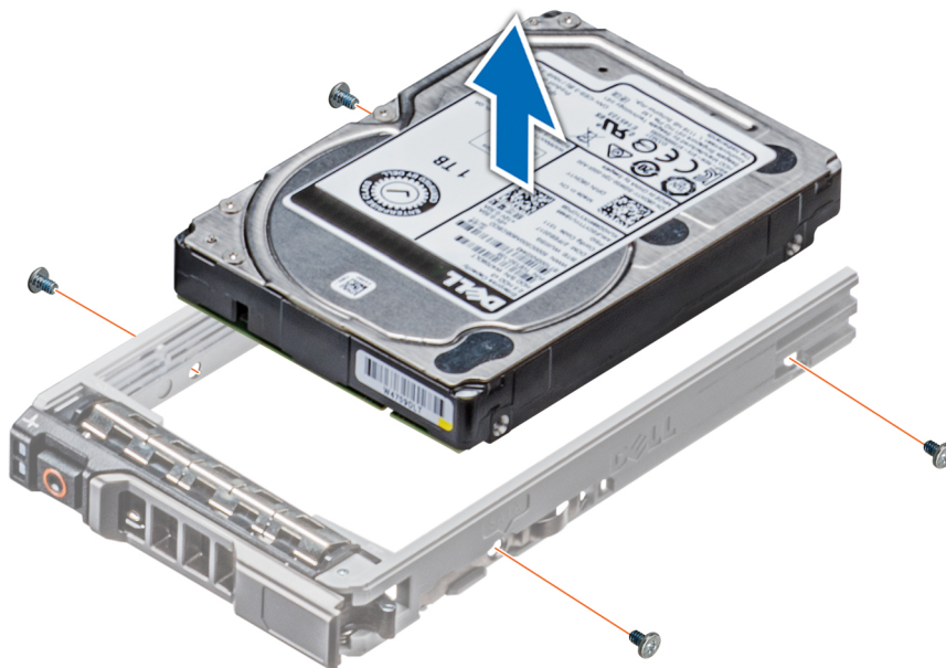
Figure 31. Retrait d'un disque dur installé de son support
