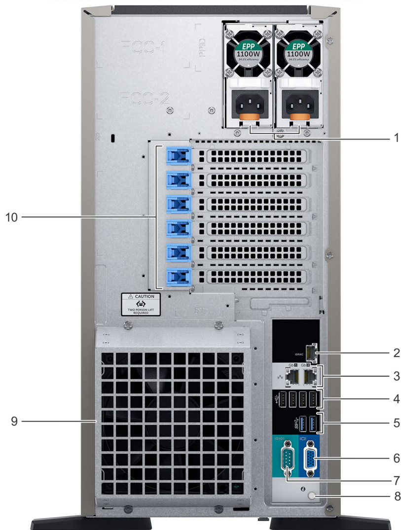
Figure 9. Vue arrière du système avec ventilateur redondant (en option)
