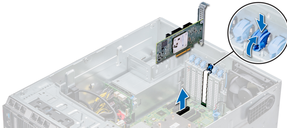
Figure 61. Retrait d'une carte d'extension
