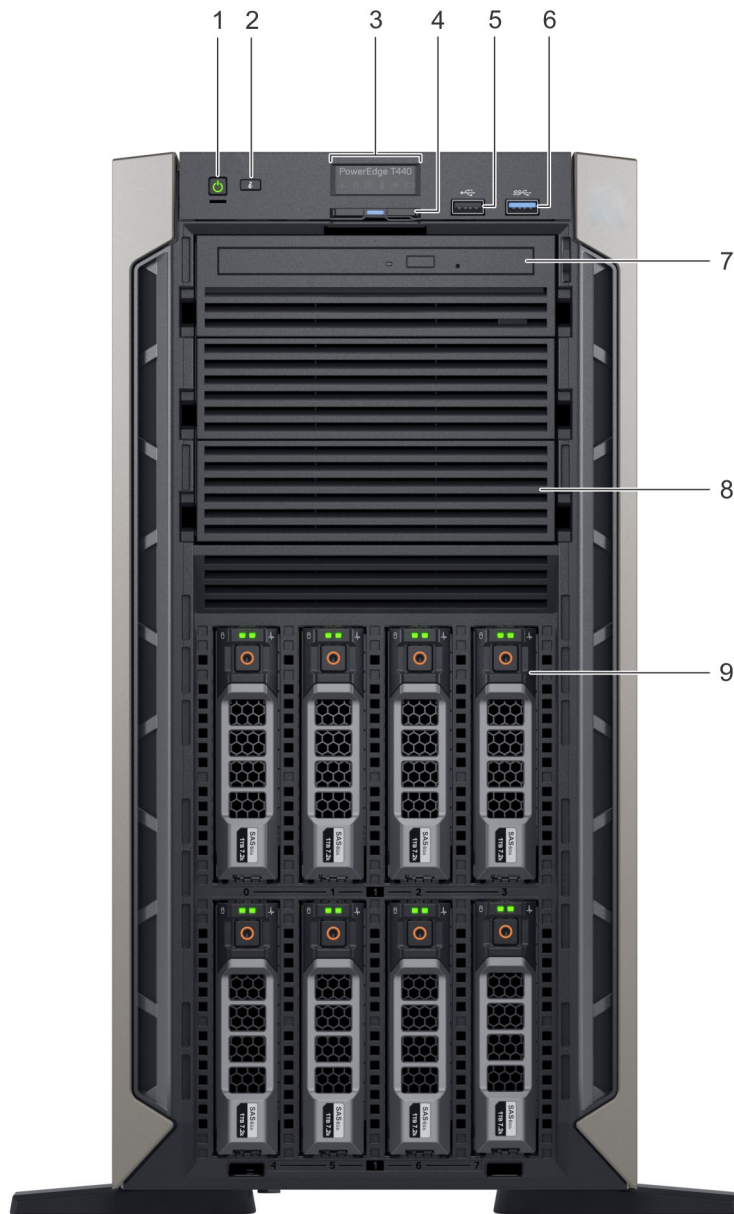
Figure 3. Vue du panneau avant d'un système à 8 disques de 3,5 pouces échangeables à chaud
