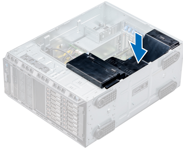
Figure 26. Installation du carénage d'aération
