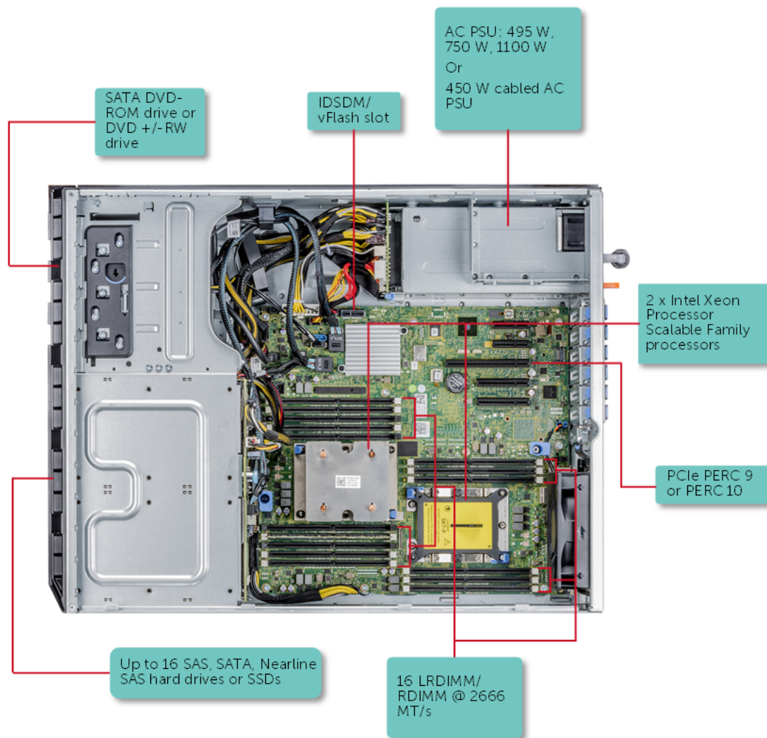
Figure 1. Configurations prises en charge par un Dell EMC PowerEdge T440 système
