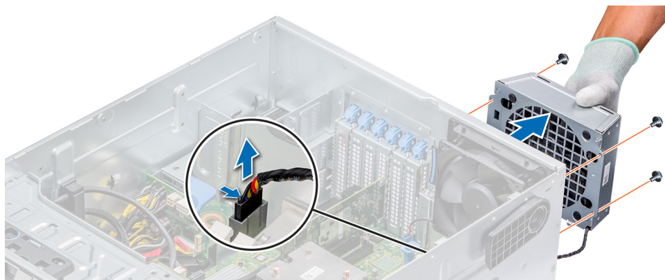
Figure 57. Retrait du ventilateur de refroidissement externe
