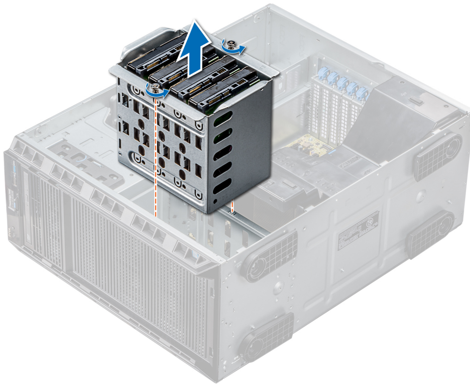
Figure 41. Retrait de la baie de disque dur interne
