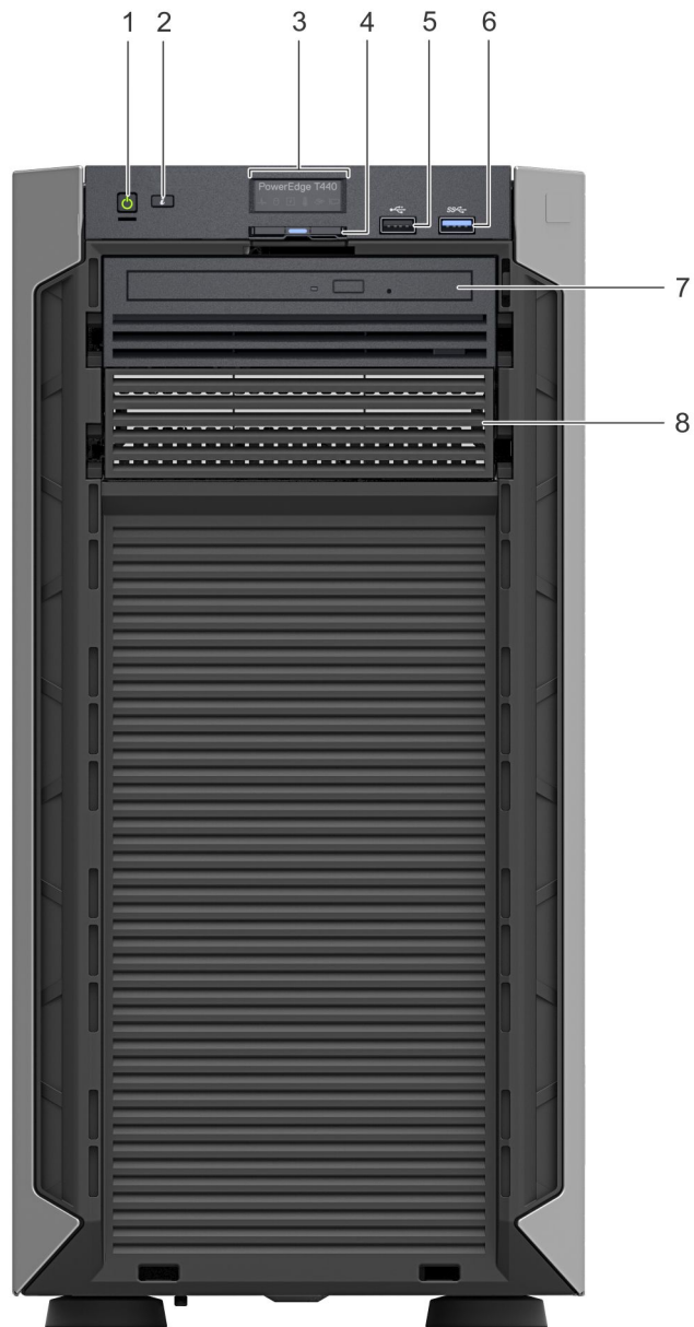
Figure 2. Vue avant d'un système de 4 disques câblés de 3,5 pouces
