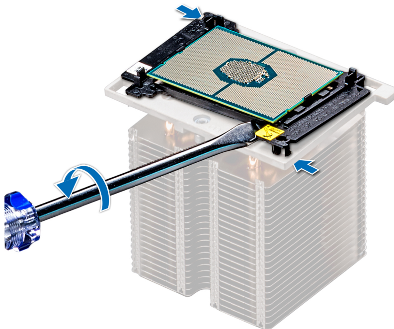
Figure 72. Pliage du support de processeur
