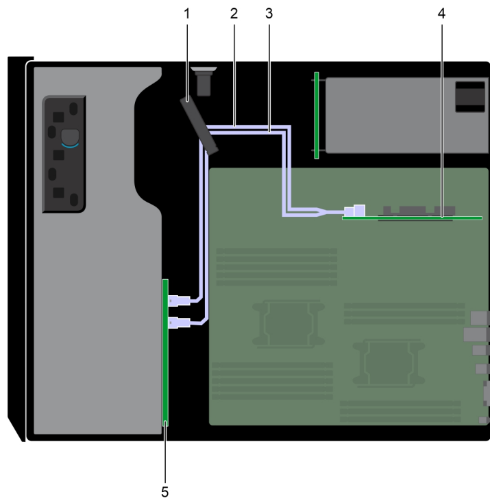
Figure 48. Acheminement des câbles : fond de panier de 16 disques de 2,5 pouces avec carte de montage PERC interne
