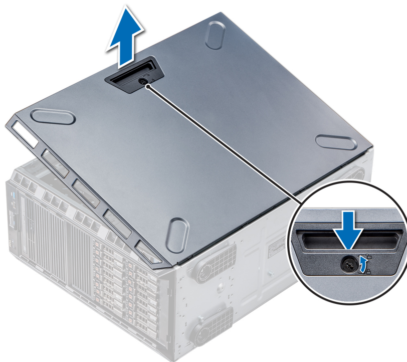
Figure 23. Retrait du capot du système
