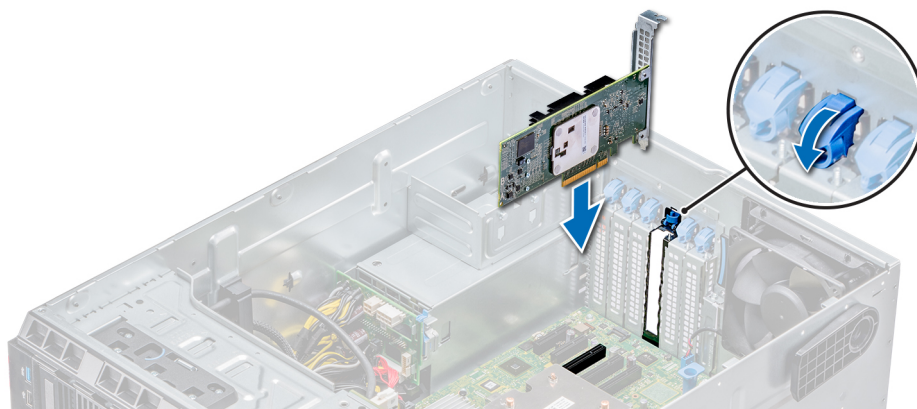
Figure 64. Installation d'une carte d'extension
