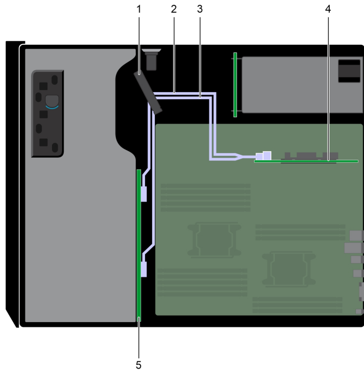
Figure 47. Acheminement des câbles : fond de panier de 8 disques de 3,5 pouces avec carte de montage PERC interne
