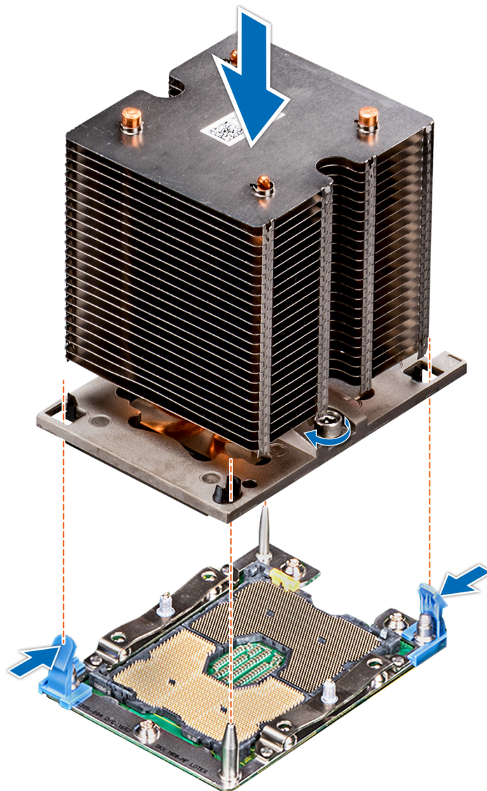
Figure 77. Installation d'un module de processeur et de dissipateur de chaleur
