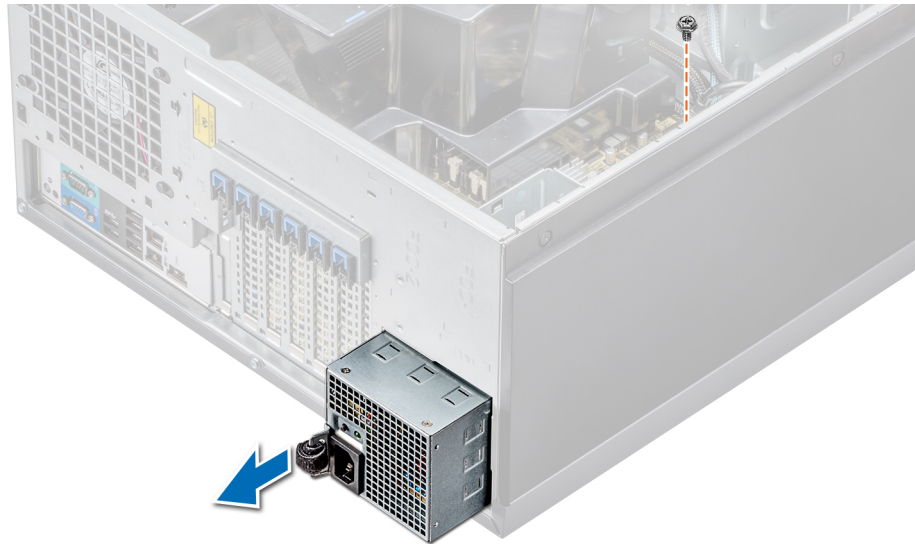
Figure 82. Retrait d'un bloc d'alimentation câblé
