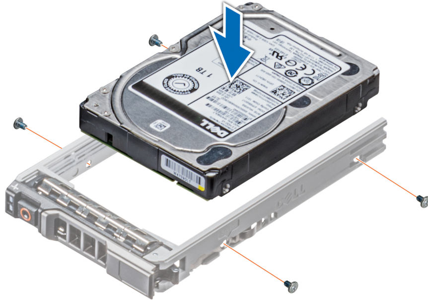
Figure 32. Installation d'un disque dans son support
