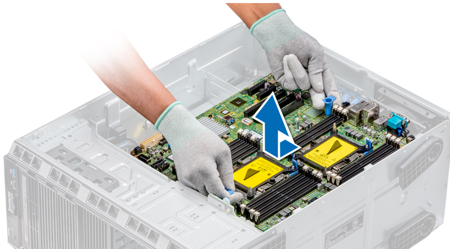
Figure 92. Retrait de la carte système
