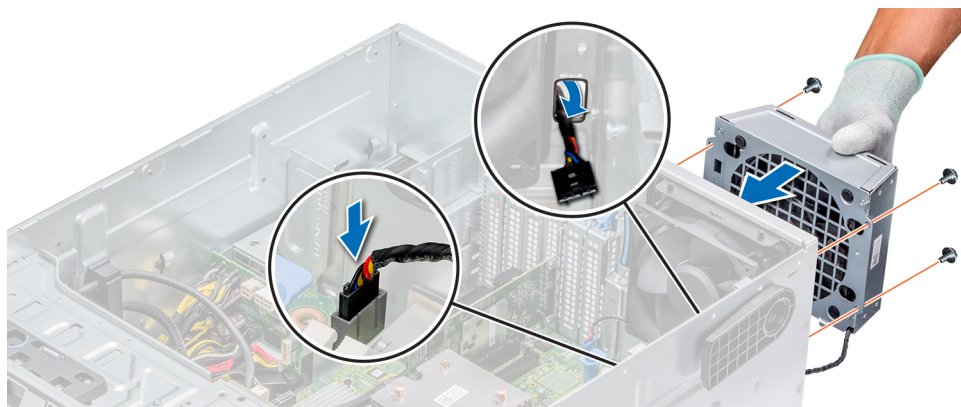
Figure 58. Installation du ventilateur de refroidissement externe
