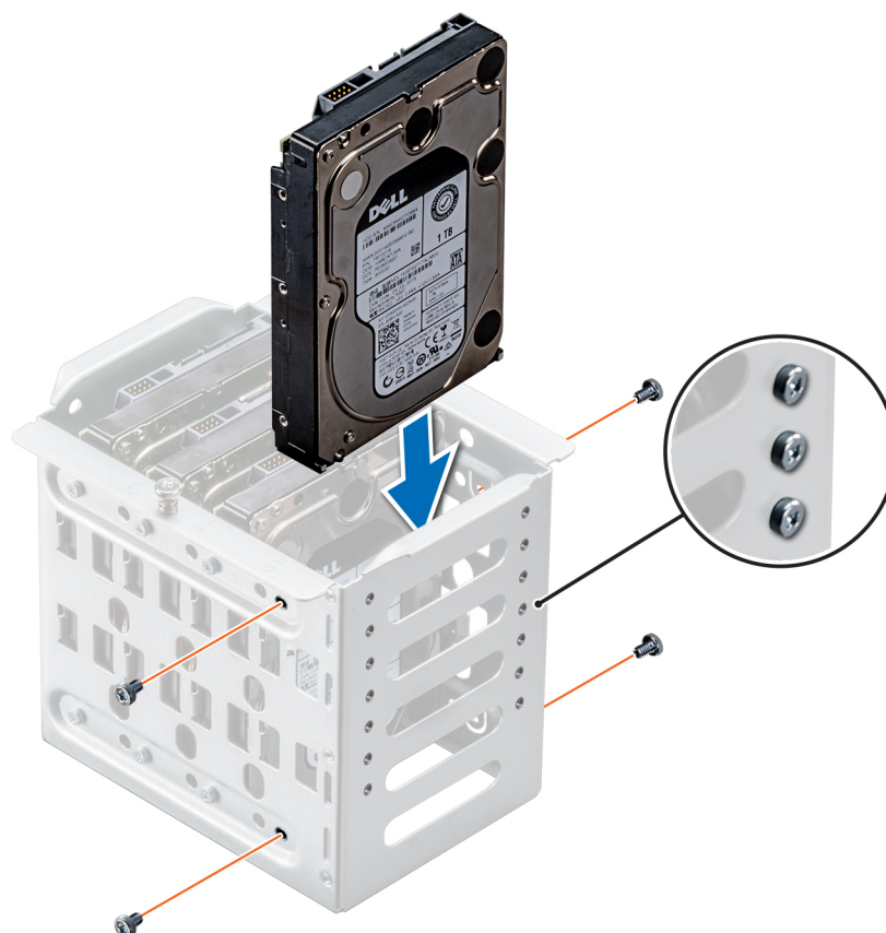
Figure 44. Installation d'un disque câblé
