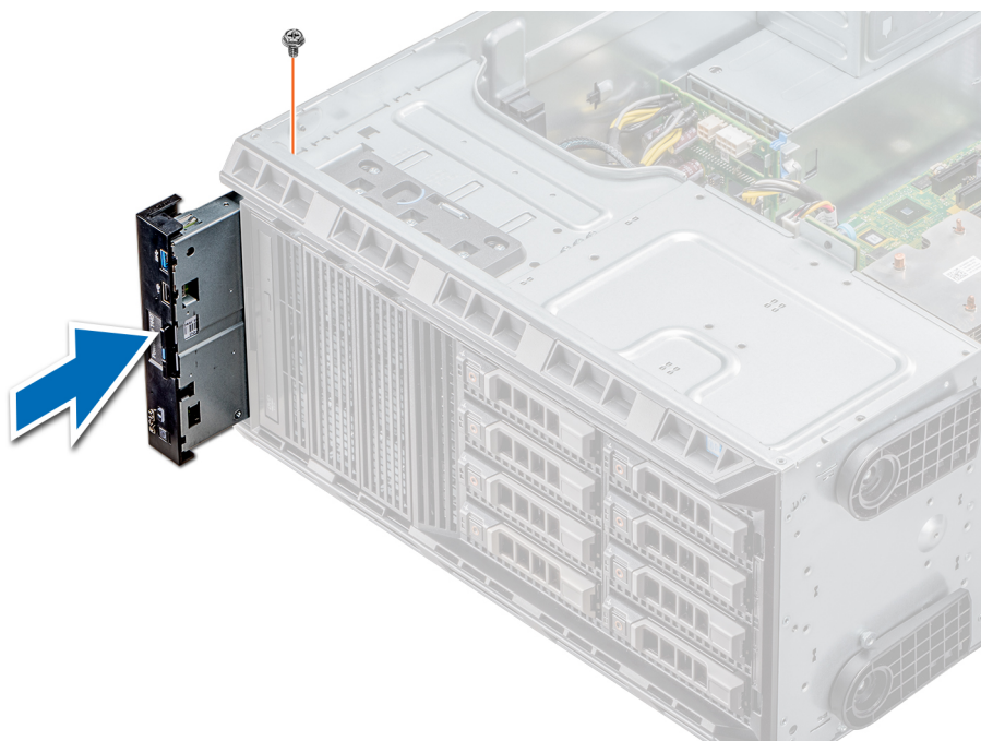
Figure 90. Installation de l'assemblage du panneau de commande
