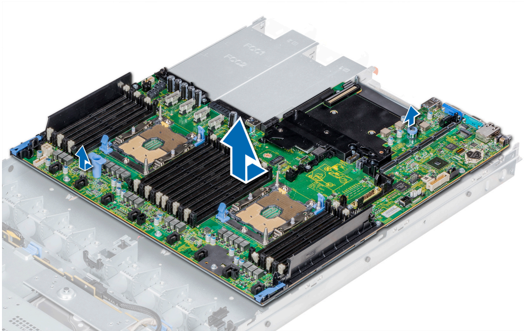
Ilustración 116. Extracción de la tarjeta madre
