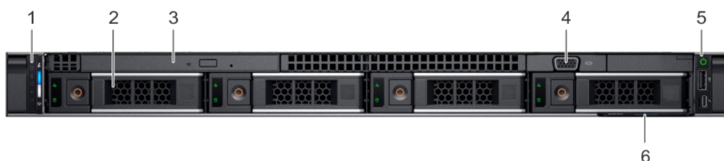
Figure 3. Vue avant d'un système à 4 disques de 3,5 pouces
