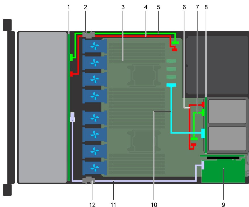
Figure 94. Routage des câbles : fond de panier de 4 disques de 3,5 pouces et fond de panier de 2 disques arrière de 2,5 pouces avec NVMe
