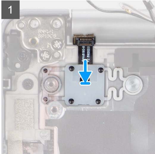
1x M2x2.5
