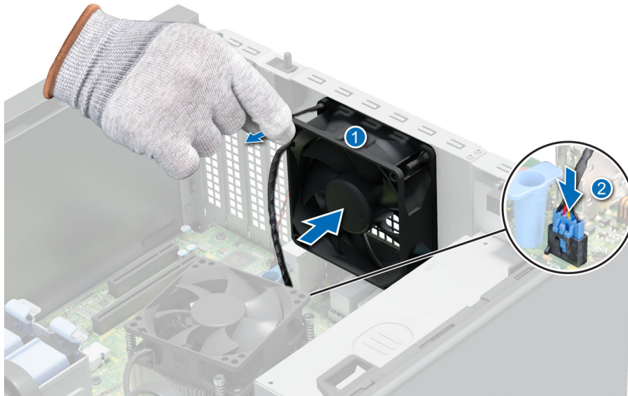
Figure 33. Installation d'un ventilateur
