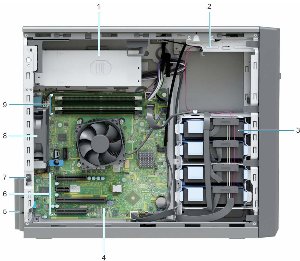
Figure 3. À l'intérieur du système
