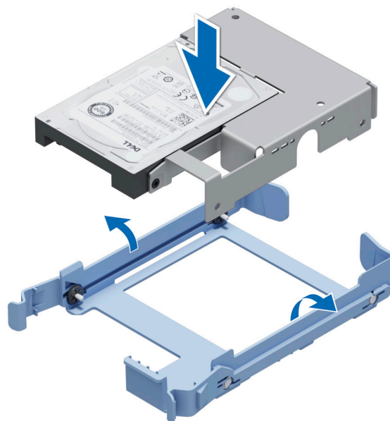
Figure 19. Installation d'un adaptateur de disque de 3,5 pouces dans un support de disque de 3,5 pouces
