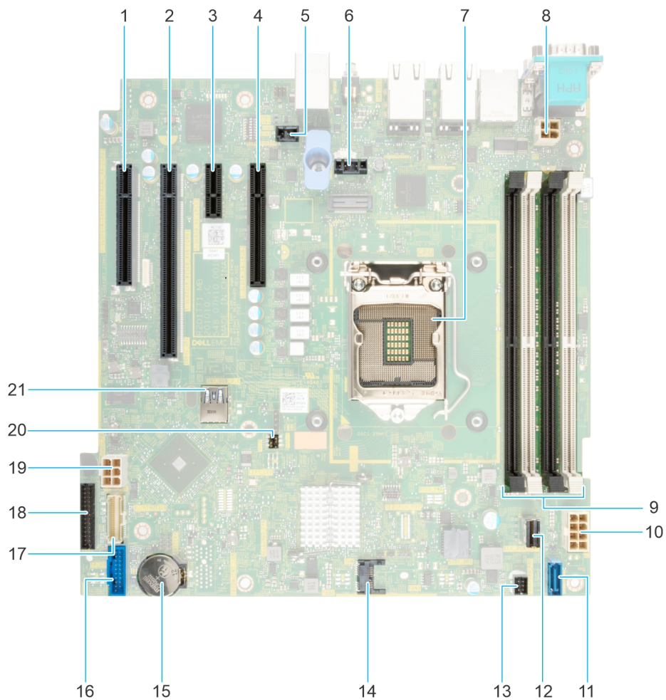
Figure 63. Connecteurs et cavaliers de la carte système
