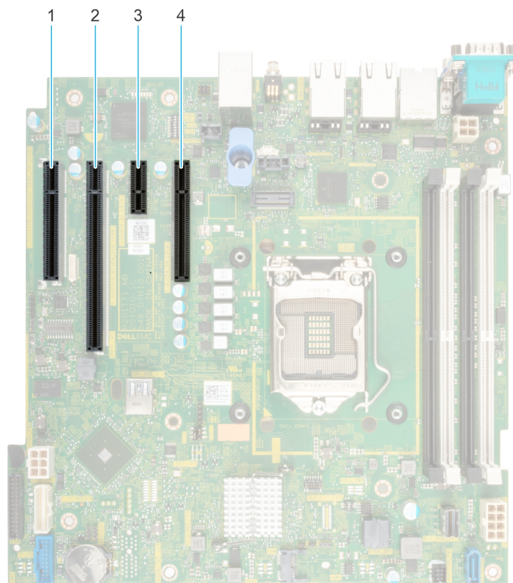
Abbildung 36. Erweiterungskarten-Steckplätze
