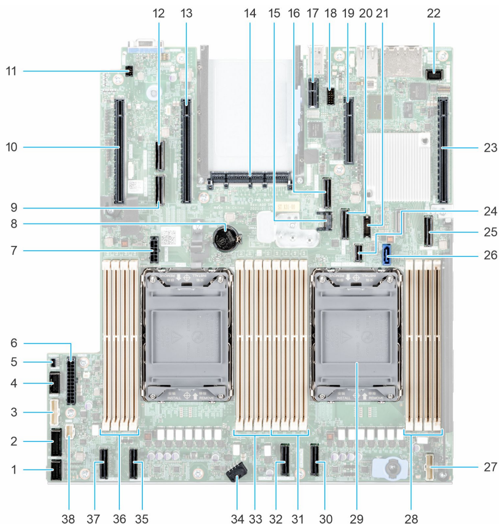
Ilustración 179. Puentes y conectores de la tarjeta madre
