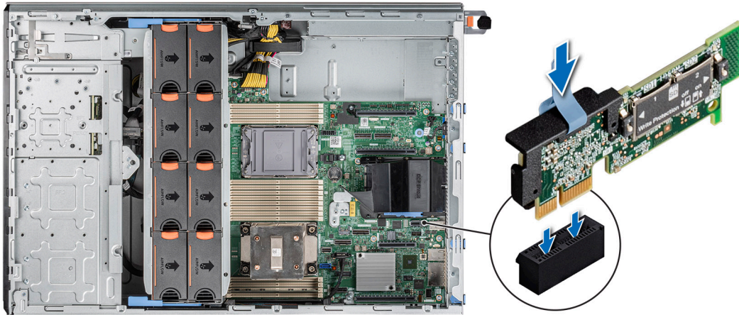
Ilustración 125. Instalación del módulo IDSDM
