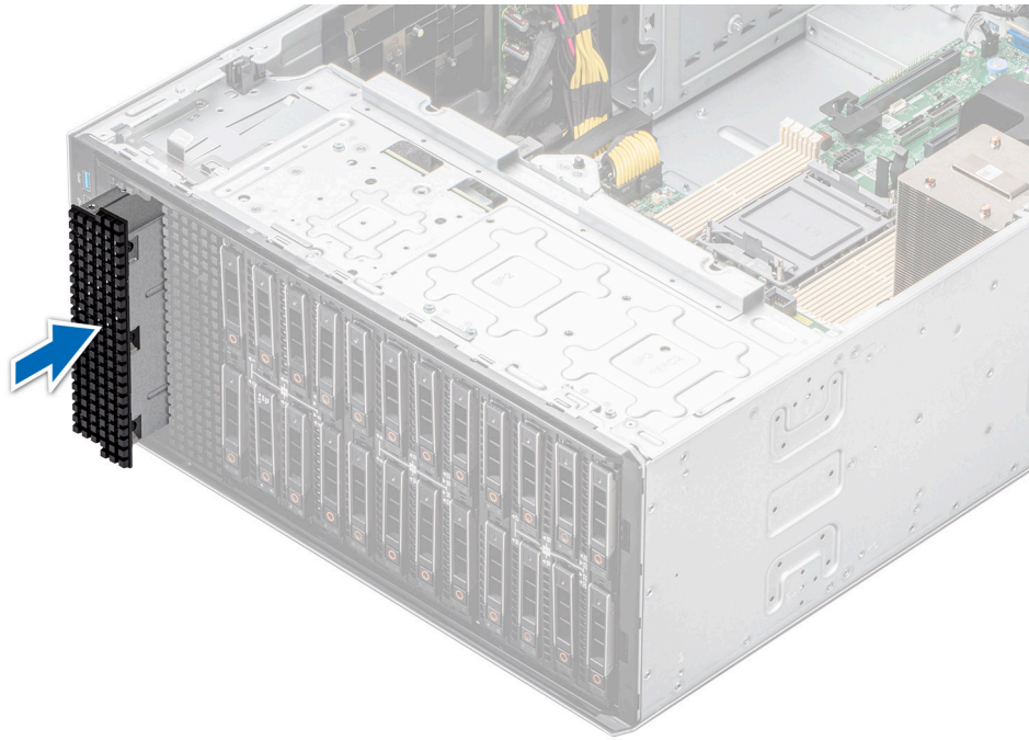
Ilustración 98. Instalación de la unidad de respaldo en cinta de relleno
