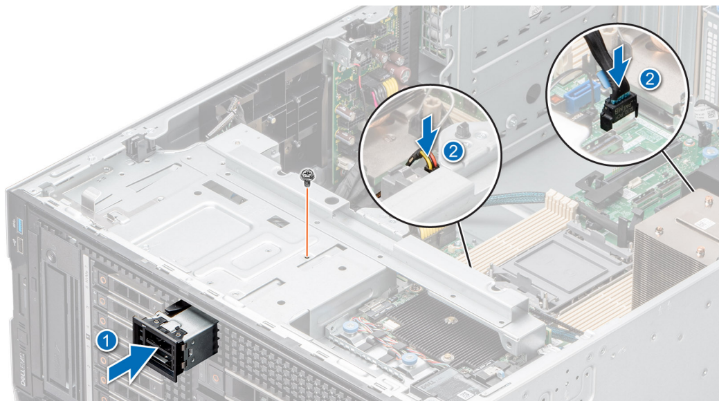
Ilustración 113. Instalación del módulo S2 de BOSS
