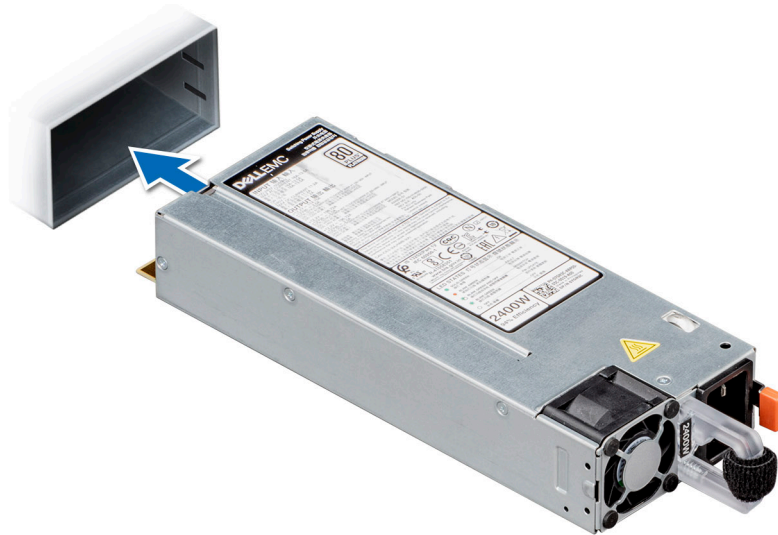
Ilustración 172. Instalación de una fuente de alimentación de 86 mm
