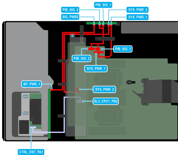
Ilustración 84. Enrutamiento de cables: 8 SAS de 3,5 pulgadas
