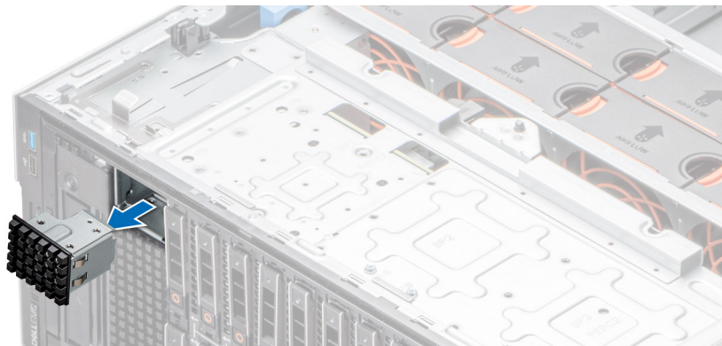
Ilustración 111. Extracción del módulo de Boot Optimized Storage Subsystem S2 de relleno
