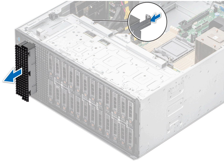
Ilustración 97. Extracción de la unidad de respaldo en cinta de relleno
