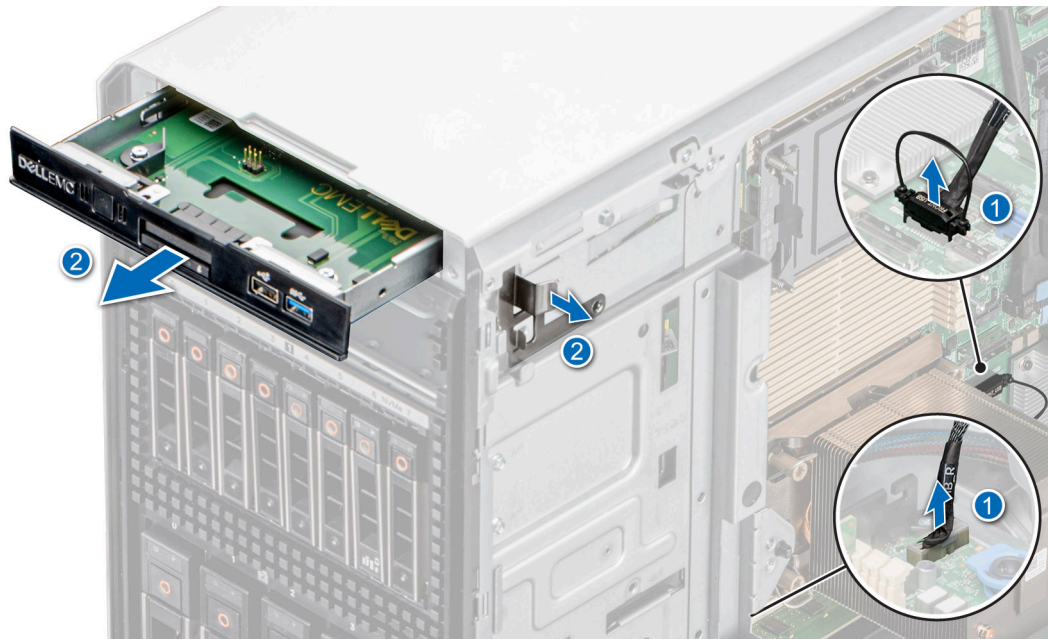
Ilustración 101. Extracción del módulo de I/O frontal para la configuración básica
