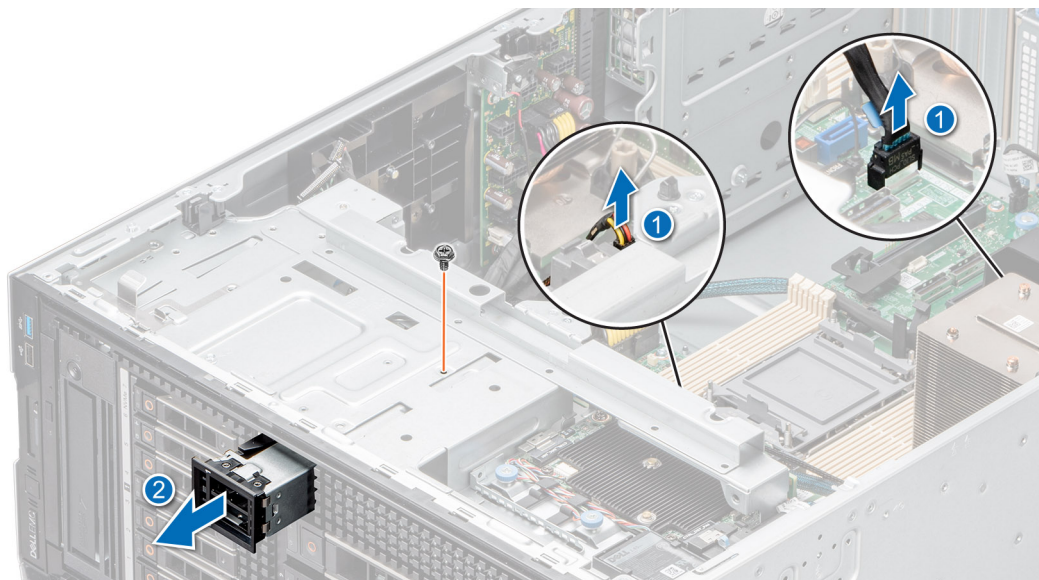
Ilustración 109. Extracción del módulo S2 de BOSS
