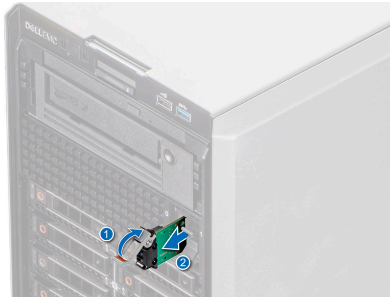
Ilustración 114. Extracción del portatarjetas de tarjeta de BOSS S2
