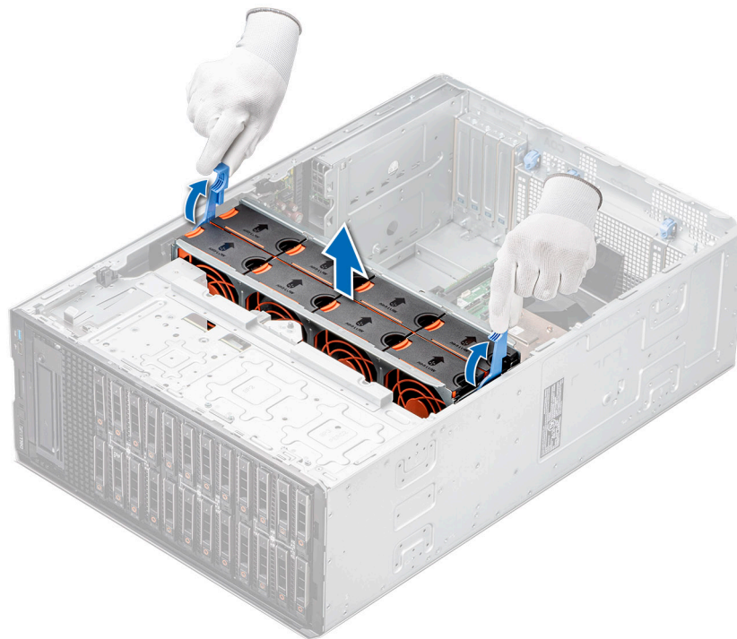
Ilustración 37. Extracción del compartimento del ventilador de refrigeración
