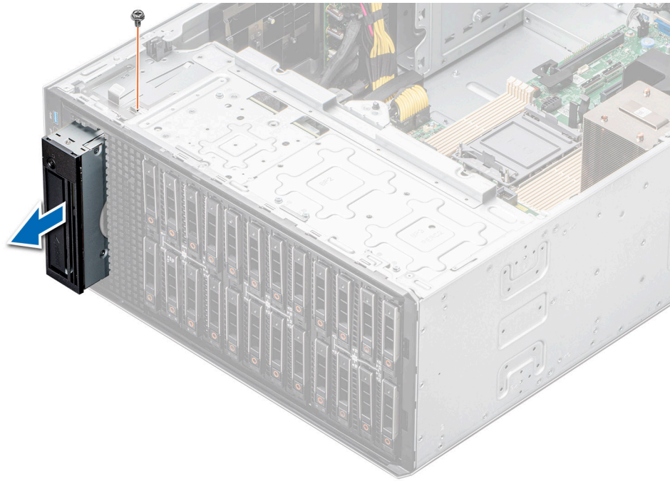
Ilustración 99. Extracción de la unidad de respaldo en cinta
