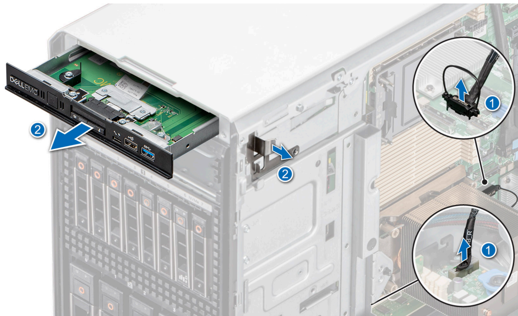
Ilustración 102. Extracción del módulo de I/O frontal para la configuración de gama superior
