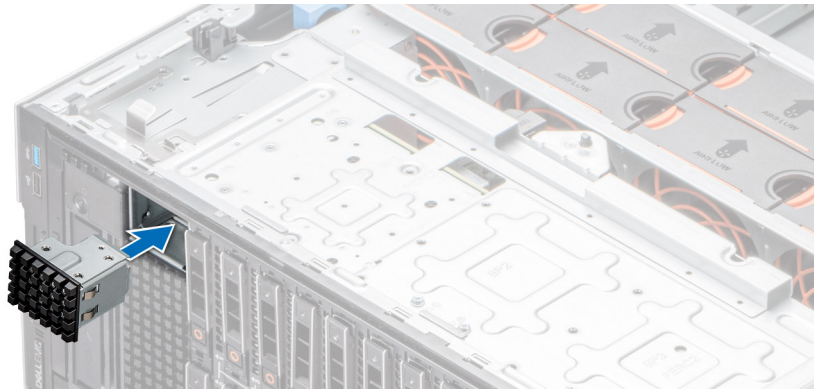
Ilustración 110. Instalación del módulo de Boot Optimized Storage Subsystem S2 de relleno
