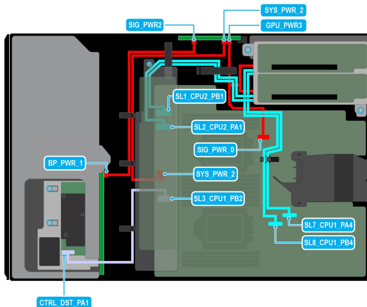
Ilustración 87. Enrutamiento de cables: 8 SAS de 3,5 pulgadas con dos soportes verticales para la GPU
