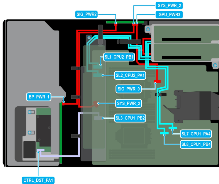
Ilustración 89. Enrutamiento de cables: 8 SAS de 3,5 pulgadas con dos soportes verticales para la GPU
