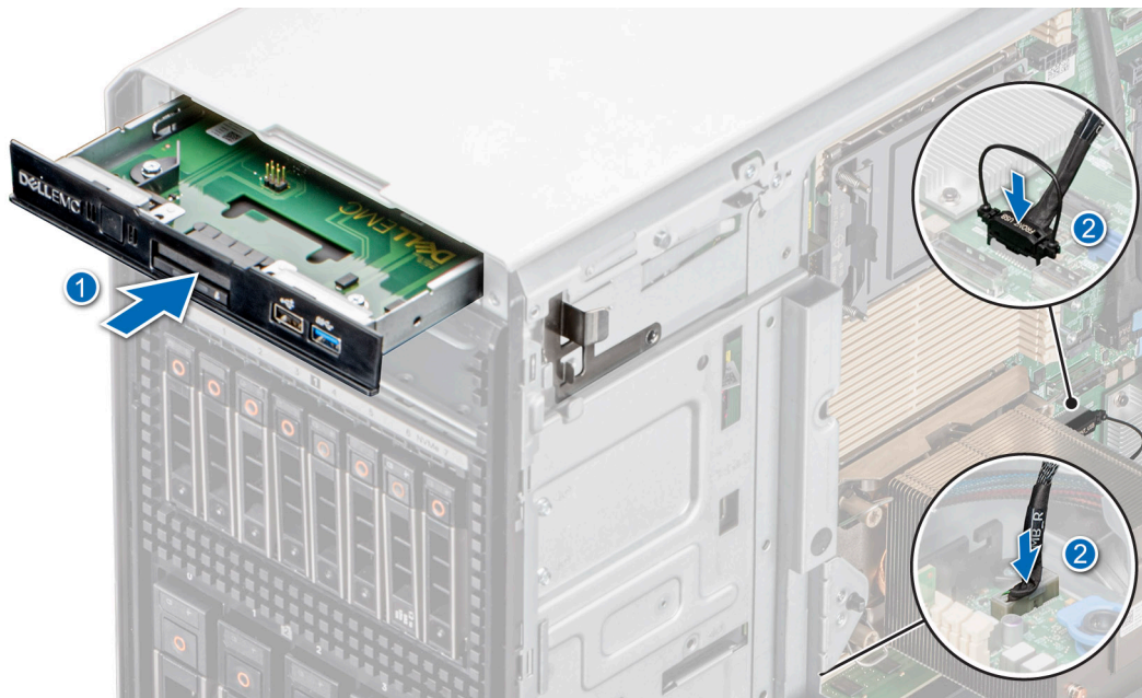
Ilustración 105. Instalación del módulo de I/O frontal para la configuración básica
