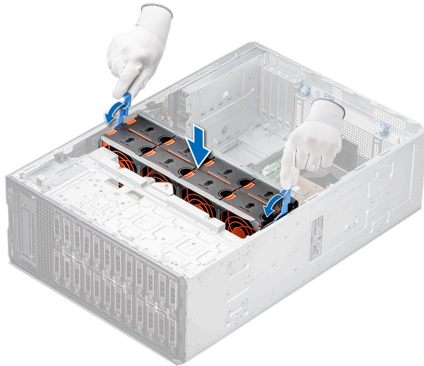
Ilustración 40. Instalación del compartimento del ventilador de refrigeración
