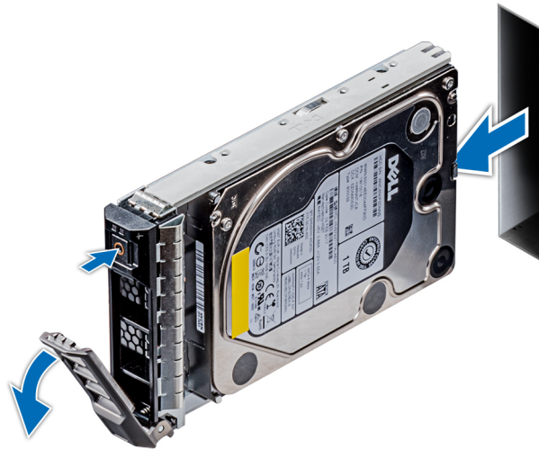
Ilustración 50. Extracción de un portaunidades
