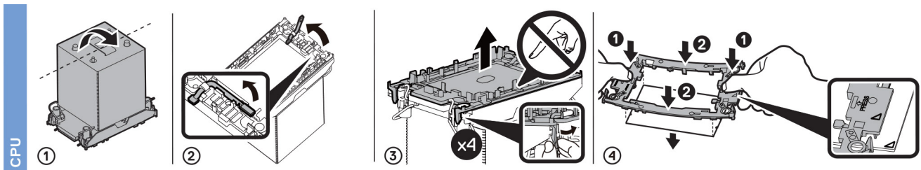
Ilustración 23. Procesador
