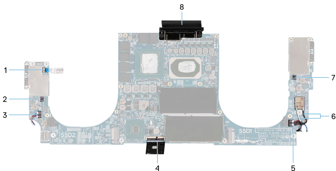
Afbeelding 2. Systeemkaartconnectoren
