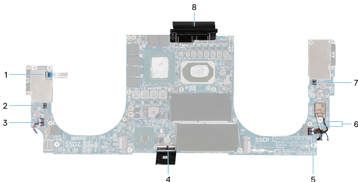
Afbeelding 1. Systeemkaartconnectoren
