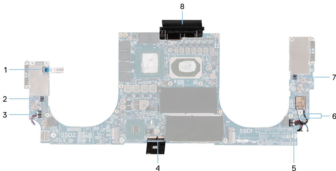
Afbeelding 1. Systeemkaartkabels
