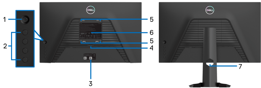
Vue arrière sans pied du moniteur
