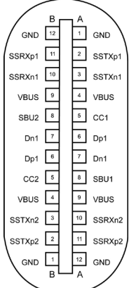
USB Type-C receptacle
