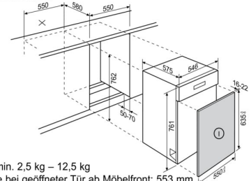
GA55LI/GLI/SLI
