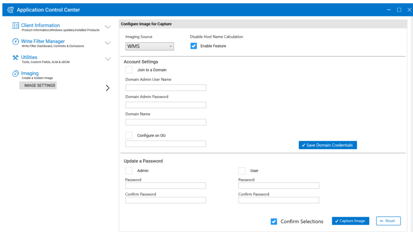
Figure 8. Confirmer une image pour la capture dans Application Control Center
