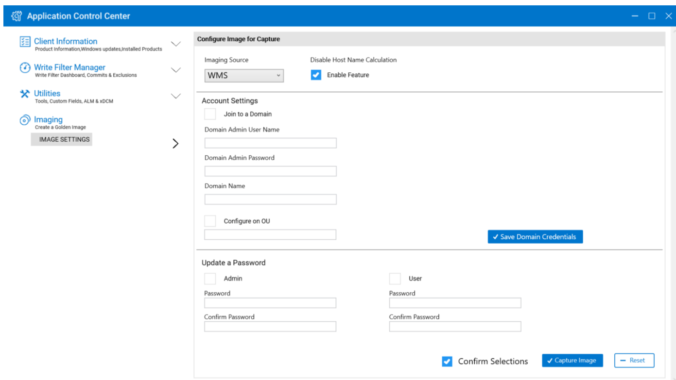
Figure 5. Confirmer une image pour la capture dans Application Control Center
