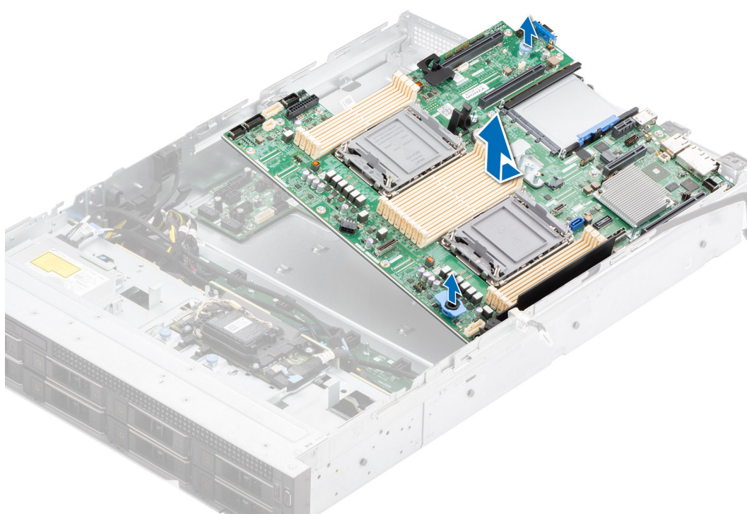
Ilustración 106. Extracción de la placa base
