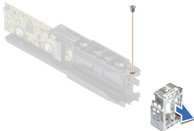
Ilustración 79. Extracción de la cubierta de BOSS
