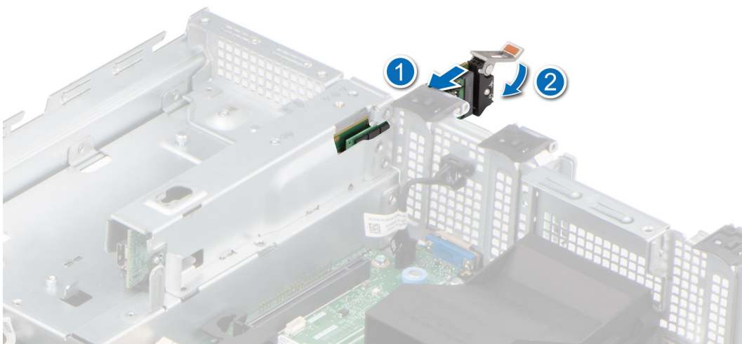
Ilustración 85. Instalación del portaunidades de la tarjeta Boot Optimized Storage Subsystem S2
