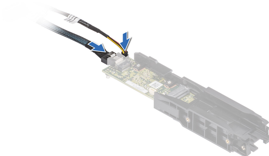
Ilustración 81. Conexión del cable de alimentación y el cable de señal de BOSS al módulo BOSS S2
