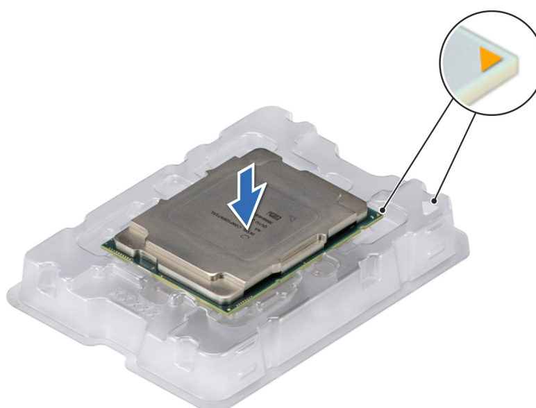
Ilustración 58. Alineación de las marcas de la pata 1 del procesador con la bandeja
