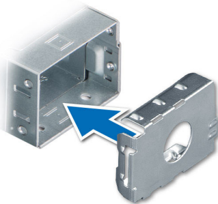
Ilustración 99. Instalación de una fuente de alimentación de relleno
