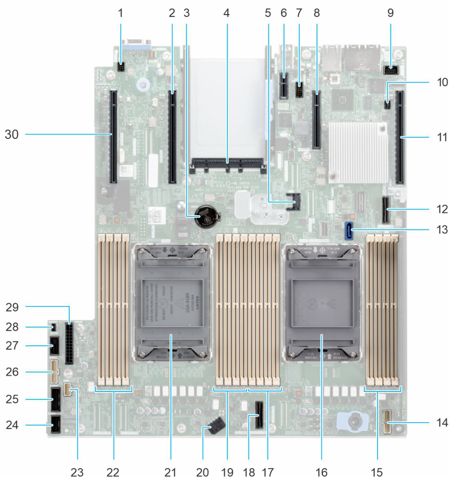
Ilustración 115. Puentes y conectores de la tarjeta madre
