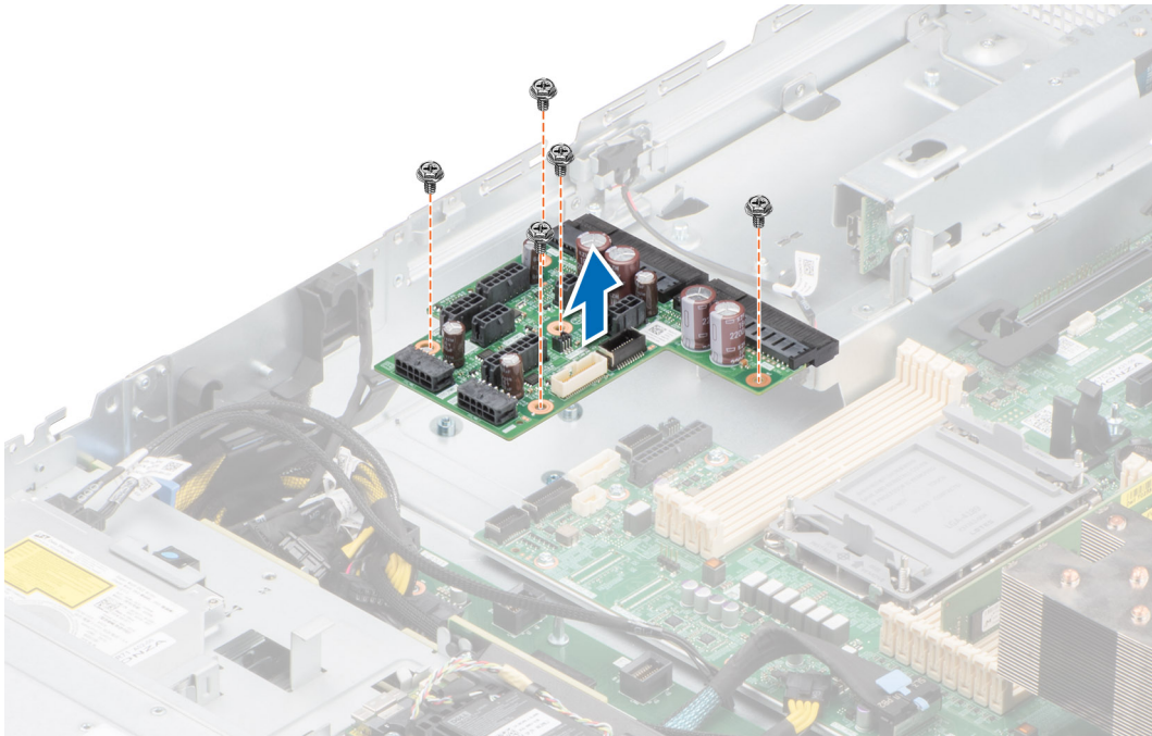
Ilustración 102. Extracción de la tarjeta mediadora de alimentación
