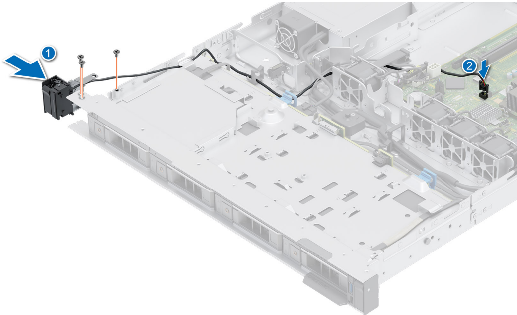
Abbildung 75. Installieren des linken Bedienfelds
