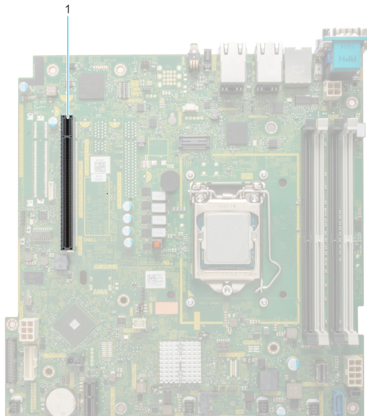
Abbildung 48. Erweiterungskarten-Steckplätze
