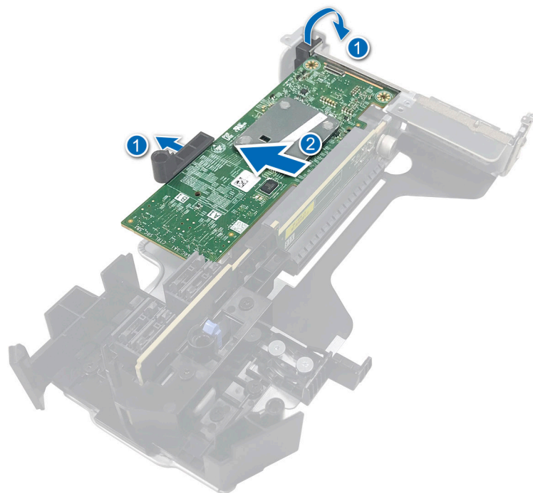
Figure 19. Retrait de l'Adaptateur HBA350i
