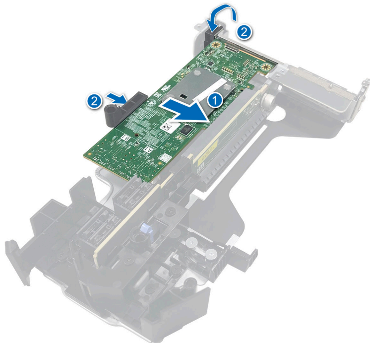
Figure 20. Installation de l'Adaptateur Dell HBA350i
