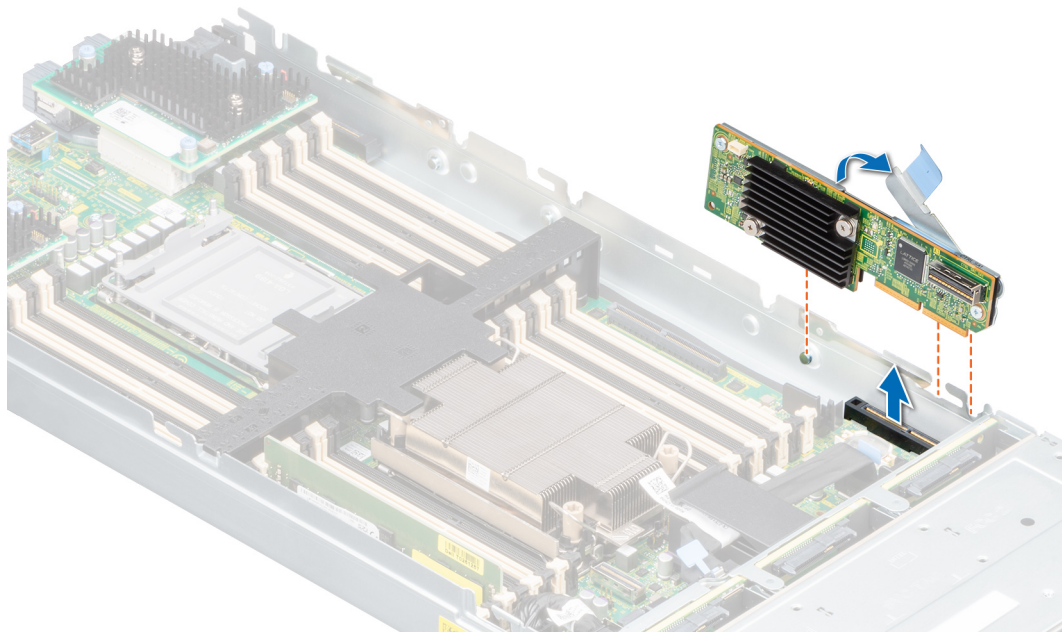
Figure 17. Retrait de la Dell HBA350i MX
