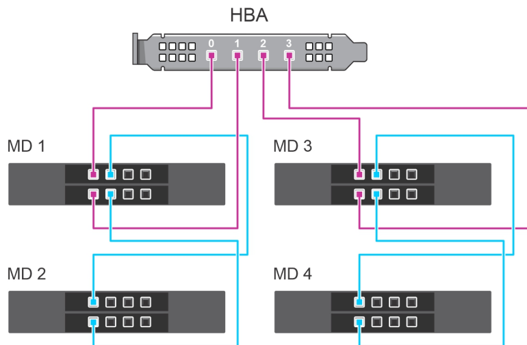
Figure 15. Configuration multichemins : câblage de Adaptateur HBA355e avec les boîtiers MD1420 et MD1400
