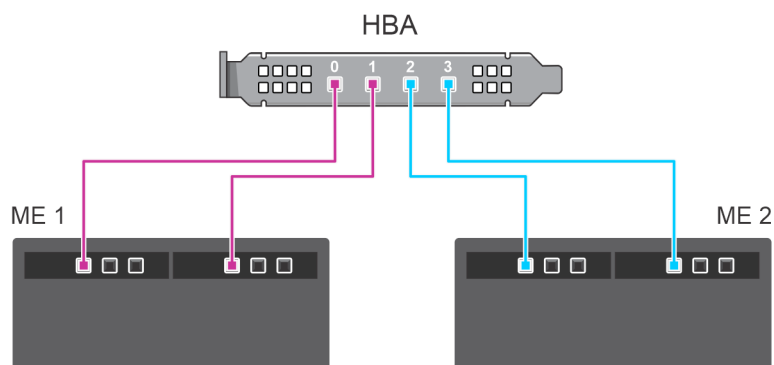
Figure 16. Configuration multicchemins : câblage de Adaptateur HBA355e avec les boîtiers ME484
