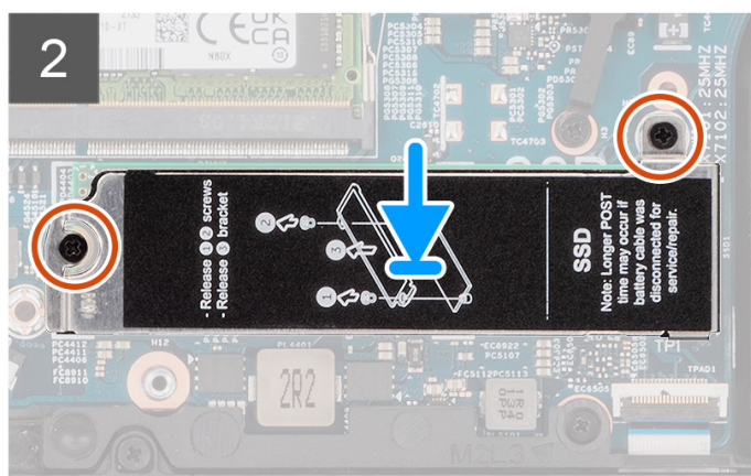
איור 4. כונן Solid-State מסוג M.2 2280 עם תושבת
