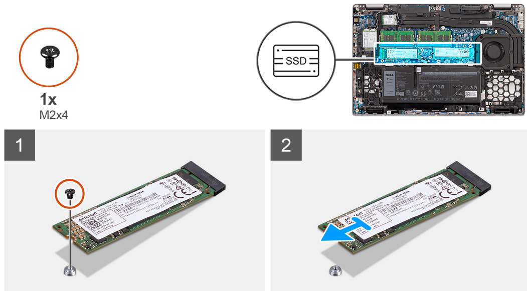
איור 1. כונן Solid-State מסוג M.2 2280 ללא תושבת
